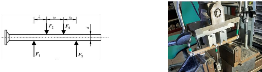
FIGURE 2. Dispositif expérimental pour essais de flexion sur chevilles circulaires en chêne
