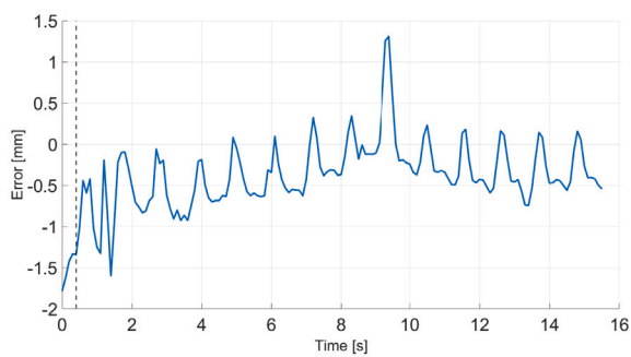
(d) Error on layer with 38 [mm] width.
