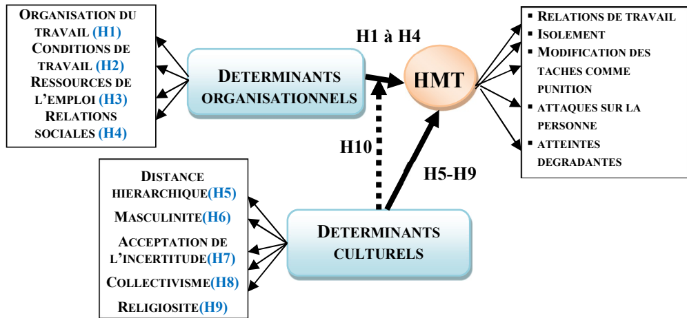
Figure 1 : Modèle conceptuel
