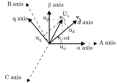
Fig. 3. abc and dq frame in Park transformation
