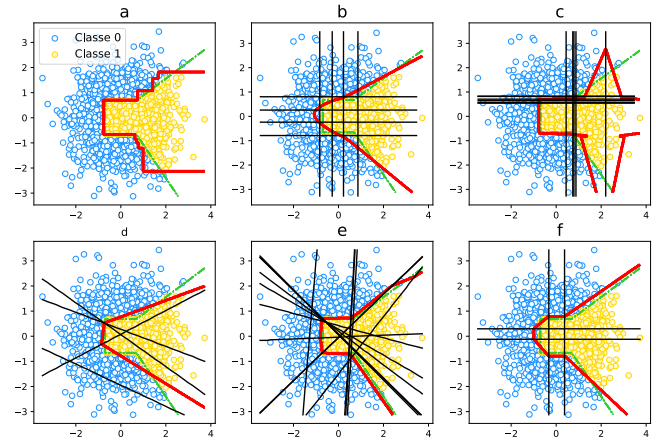
FIGURE 2 – Résultats sur données simulées : a) DT, b) RL SNC, c) MARS avec M = 10 , d) RN avec p = 4 dans (5), e) RN avec p = 30 dans (5), f) RN-MARS. Légende : frontière idéale en vert, frontière estimée en rouge, segmentation en noir.
