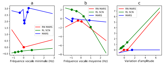
FIGURE 3 – Splines estimées sur les données réelles : a) Fréquence vocale minimale, b) Fréquence vocale moyenne, c) Variation d’amplitude. Légende : RN-MARS en rouge, MARS en bleu, RL SCN en vert.
