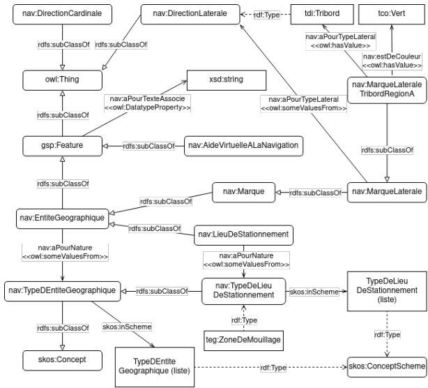
FIGURE 4 – Un extrait du graphe du modele.
