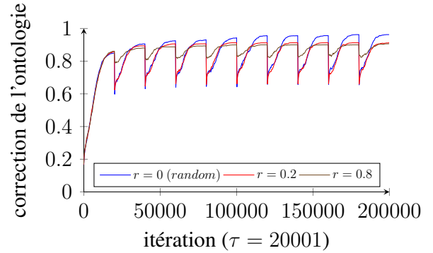
FIGURE 5 – Correction moyenne avec (rouge et marron) ou sans (bleu) transmission verticale initiale.
