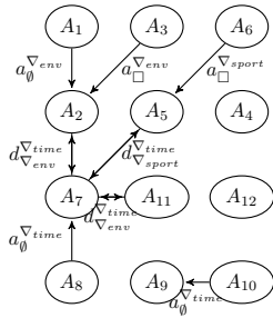
FIGURE 1 – Graphe d’argumentation
