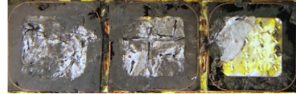
(d) Dies after dynamic avalanche destruction.
