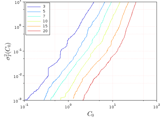
FIGURE 3 – EQM \sigma_T^2(C_0) en fonction du seuil C_0 et de l'échelle d'observation T \in \{3, 5, 7, 10, 15, 20\} .
