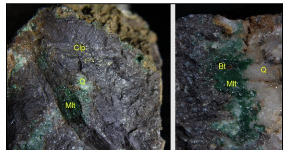
Fig.24 : fragment de minerais cuprifère collecté in situ au niveau du site d'extraction ancien O-L-M-3. Q : quartz, Clp : chalcoppyrite, Mlt : malachite, Bt : bornite.
