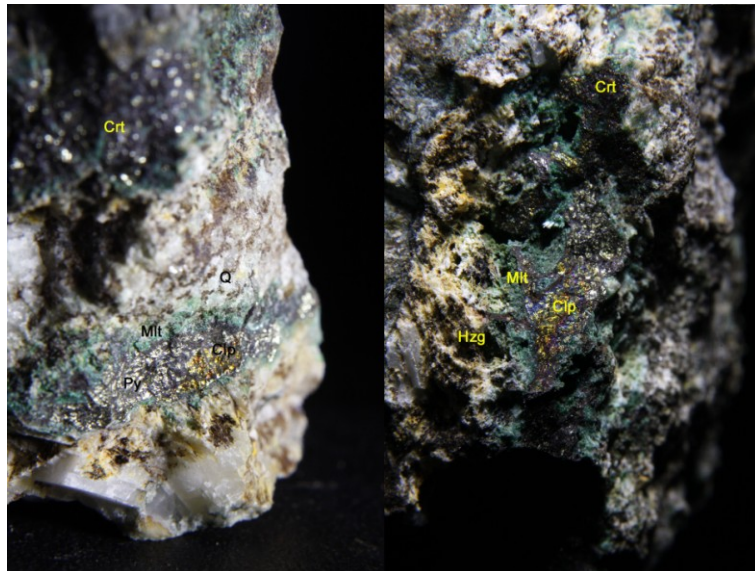
Fig. 35 : exemples de minerais cuprifères minéralisés dans le site O-S-M-1. Q : quartz, Clp : chalcopyrite, Mlt : malachite, Cr : chromite, Py : pyrite, Hzt : harzburgite.
