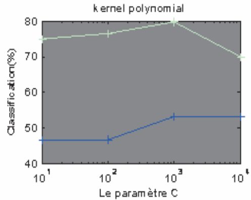
FIG. 3 : la courbe représentant le taux de classification du noyau polynomial du classifieur en fonction du paramètre C
