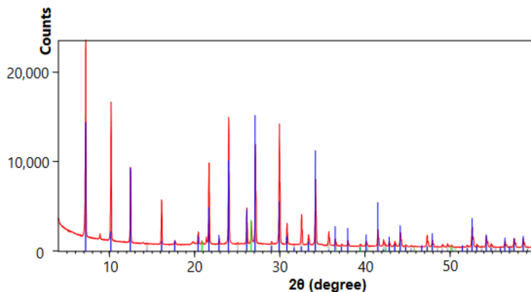
Figure 1. XRD pattern of 4AZW.
