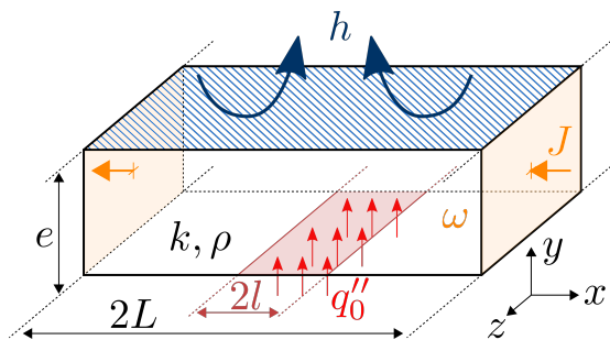
Figure 1 : Géométrie 3D dimensionnée
