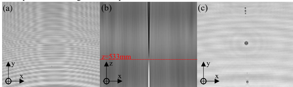
Figure 3: (a) Hologramme de perles issu de l'étirement d'un fluide viscoélastique. (b) Localisation d'une perle par étude de la carte de phase selon les axes (x,z) . (c) Restitution optimale de l'hologramme à z = 533 mm.
