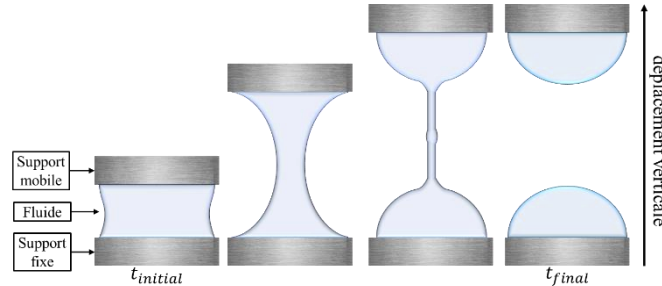
Figure 2: Schéma du dispositif CaBER pour l'étirement des fluides viscoélastiques.
