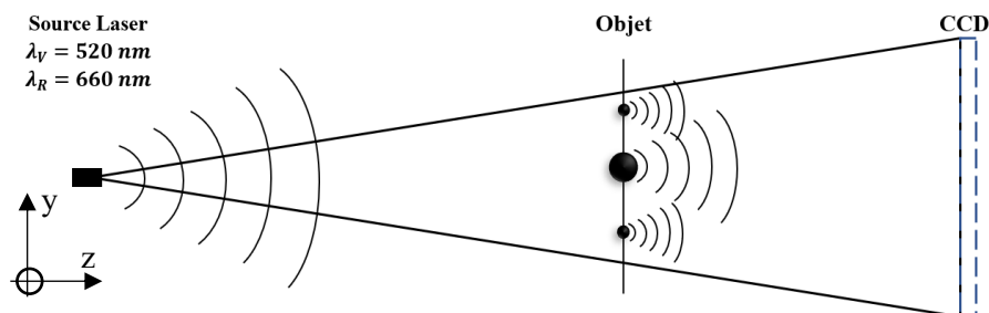
Figure 1: Dispositif expérimental pour l'enregistrement d'un hologramme de gouttelettes issues de l'étirement d'un fluide viscoélastique.
