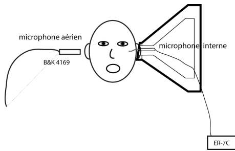
FIGURE 1 – Dispositif expérimental.
