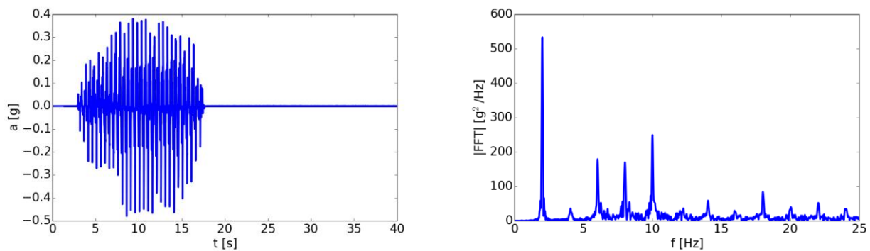
Figure 7. Signal appliqué à la base du modèle. À droite : représentation temporelle ; à gauche : représentation fréquentielle.
