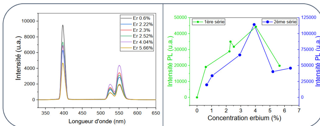
Figure 1 : Gauche, spectres d'émission montrant les signaux de SHS (400 nm) et UC-PL (525 et 550 nm) de suspensions de nanocristaux de LN dopés, excitation à 800 nm. Droite, intensité d'UC-PL détectée en fonction de la concentration molaire d'erbium insérée (deux séries différentes d'échantillons sont présentées).
