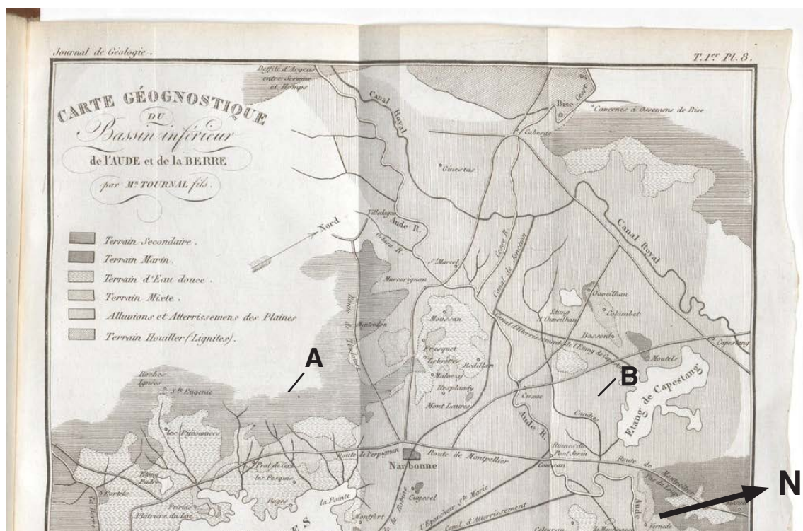
Fig. 4 – Extrait de la « Carte géognostique du Bassin inférieur de l'Aude et de la Berre » (Tournal, 1830). Localisation du « Terrain marin » : A . sud de Gruissan, au centre de l'Île Saint-Martin ; B . les Budadelles.
