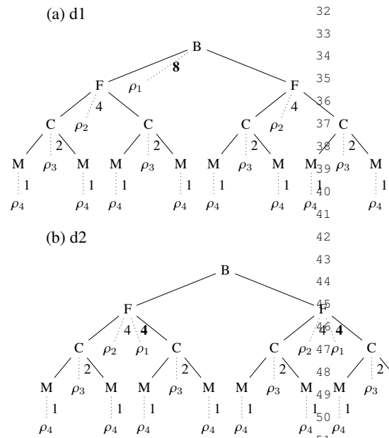
Fig. 15. d^* topologies
