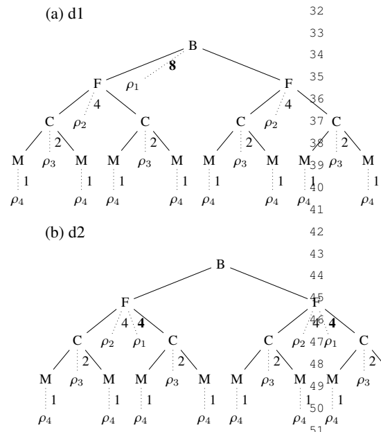
Fig. 15. d^* topologies
