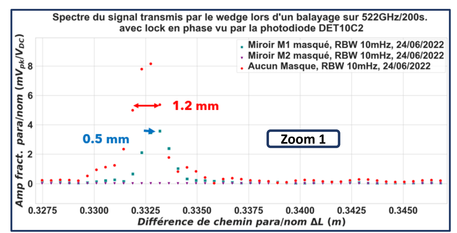
Spectre du signal du simulateur SAT lors d'un balayage en fréquence (2.61 GHz/s) du laser Echelle linéaire. Avec (bleu) et sans (rouge) masque devant les miroirs M1 et M2
