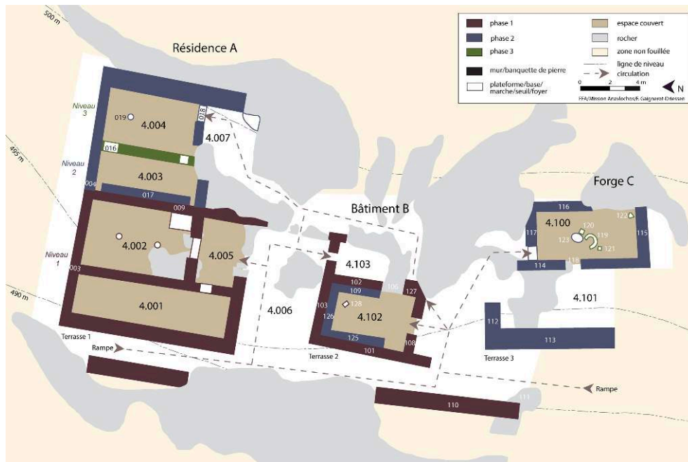
Fig. 20. Plan schématique du Quartier de la forge.
