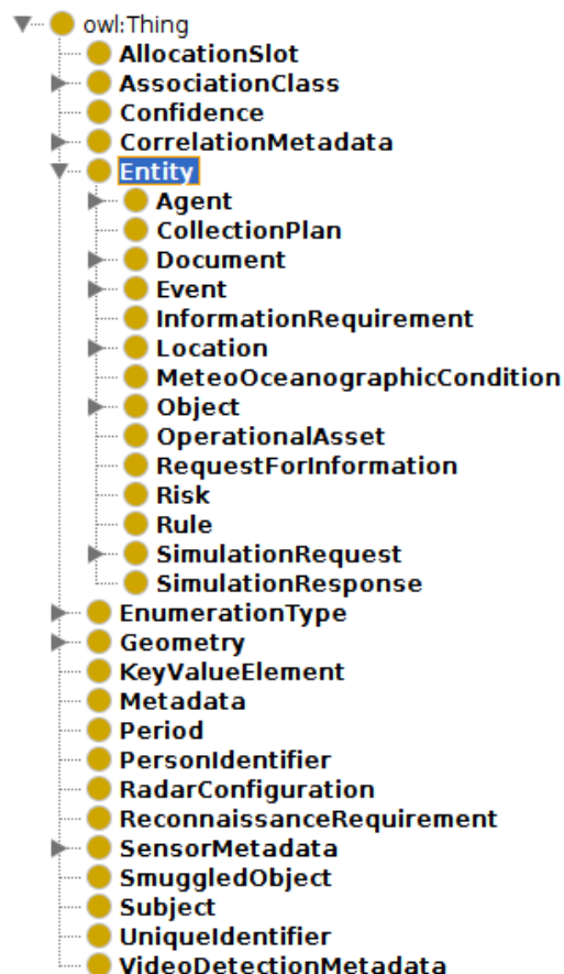
FIGURE 2 – Hiérarchie des concepts principaux d'eCISE-OWL.
