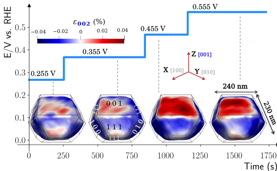
Figure 1 : Influence du potentiel de l'électrode sur la composante normale du tenseur de déformation dans la direction [001].
