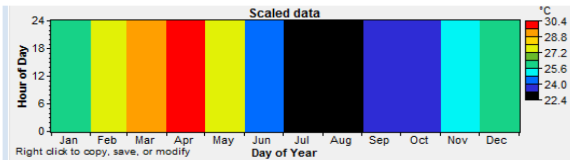
Figure N ° 7 : DMap de la température ambiante à Mamou
