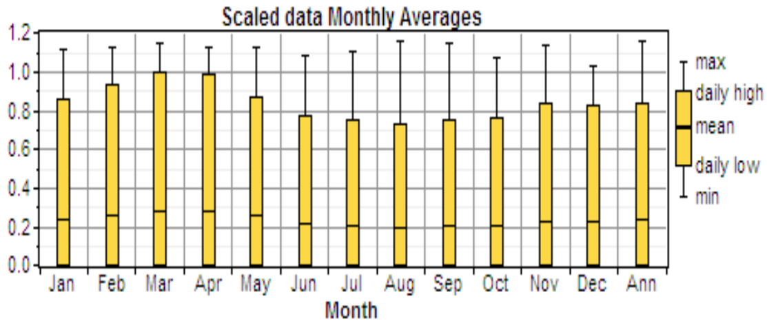
Figure N° 3 : Profil de l'éclairage moyen mensuel à Mamou
