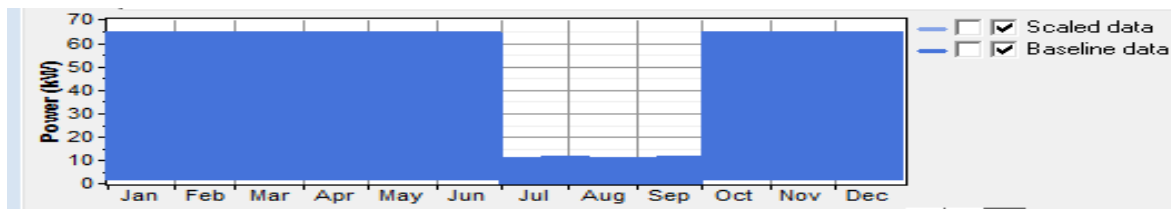
Figure N°12 : Profil annuel des charges de l'IST-Mamou
