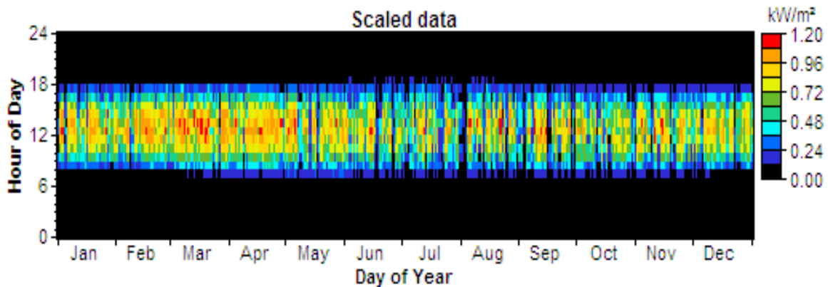
Figure N° 4 : DMAP de l'éclairage à Mamou
