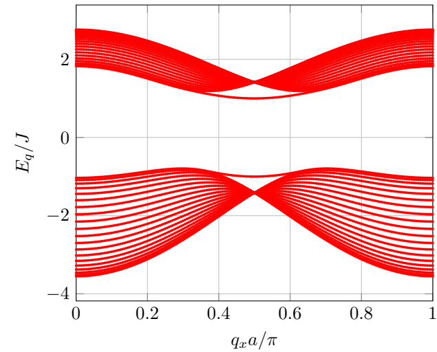
FIGURE V.26. Réseau "mur de briques" avec un ruban de n_y = 20 lignes, cas non topologique : J' = J/10 , \Delta = J , \phi_0 = 0 . Haut : conditions aux limites périodiques selon y . Bas : conditions aux limites ouvertes.
