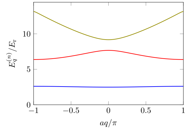
FIGURE I.7. Les trois premières bandes d'énergie ( n = 0, 1, 2 ) pour le potentiel sinusoidal V(x) = V_0 \sin^2(\pi x/a) , tracées ici pour V_0 = 8E_r , avec l'énergie de recul E_r définie par E_r = \pi^2 \hbar^2 / (2ma^2) .
