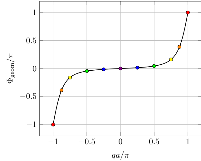
FIGURE III.23. Phase géométrique déduite de l'angle solide sous-tendu par la trajectoire de l'état |u_{q,t}\rangle sur la sphère de Bloch au cours d'un cycle de la pompe. Cette phase géométrique varie continuellement de -\pi à +\pi quand q décrit la zone de Brillouin, ce qui entraîne la quantification du déplacement \Delta x donné en (III.44). Le code de couleurs des différents points est le même que celui de la figure III.22.
