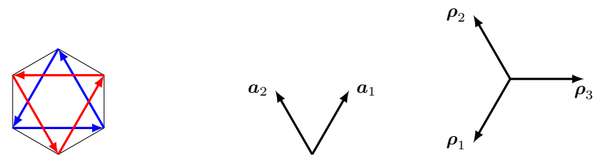
FIGURE V.3. Gauche : liens entre second voisins à l'intérieur d'un hexagone donné dans le modèle de Haldane. Droite : les vecteurs utilisés pour paramétriser les sites et les liens du réseau.
