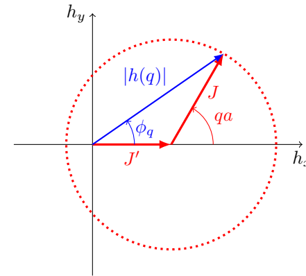
FIGURE I.15. Tracé dans le plan complexe de h(q) \equiv J' + Je^{iqa} = |h(q)| e^{i\phi_q} pour le cas J' < J . Le contour décrit par h(q) entoure l'origine et la phase \phi_q varie continument de \phi_q = -\pi à \phi_q = \pi quand q décrit la zone de Brillouin [-\pi/a, \pi/a] .
