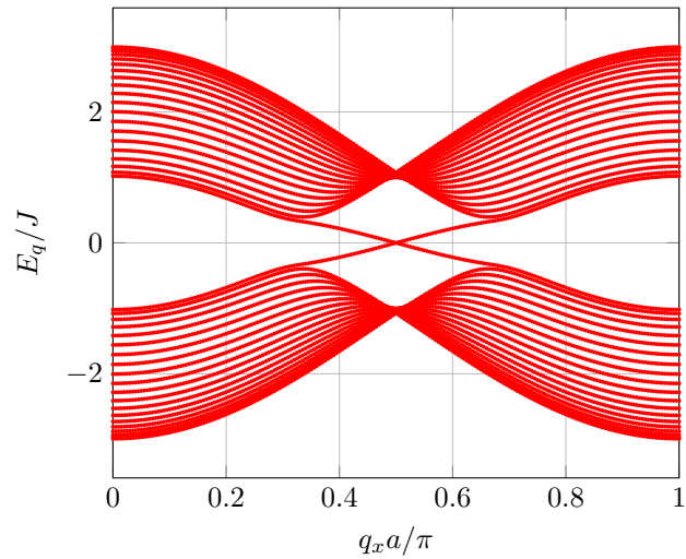
FIGURE V.25. Réseau "mur de briques" avec un ruban de n_y = 20 lignes, cas topologique : J' = J/10 , \Delta = 0 , \phi_0 = \pi/2 . Haut : conditions aux limites périodiques selon y . Bas : conditions aux limites ouvertes.
