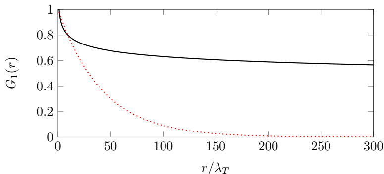
FIGURE III.7. Ligne continue noire : variation de G_1 pour une densité dans l'espace des phases \mathcal{D} = 10 pour le cas algébrique (en présence d'interactions), G_1(r) \sim (\lambda_T/r)^{1/\mathcal{D}} . Ligne pointillée rouge : cas sans interaction, G_1(r) \sim e^{-r/\ell} avec \ell = (\lambda_T/\sqrt{4\pi}) e^{\mathcal{D}/2} \approx 40 \lambda_T .
