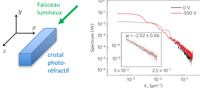
FIGURE III.6. Principe de la « condensation d'ondes classiques lumineuses » : on envoie un faisceau laser avec un certain désordre en amplitude et en phase dans un cristal photo-réfractif. Pour une longueur d'interaction suffisamment grande, l'évolution non-linéaire du champ lumineux conduit à une distribution quasi-thermique des modes transverses du faisceau lumineux. Cette distribution est caractérisée par une décroissance de la population des modes comme 1/k_{\perp}^2 . Figure extraite de SUN, JIA et al. (2012).
