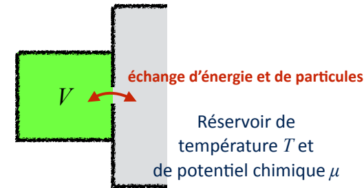
FIGURE VI.2. Ensemble grand-canonique : le système peut échanger de l'énergie et des particules avec un réservoir, qui impose sa température T et son potentiel chimique \mu (variables intensives). Le volume du système reste fixé.
