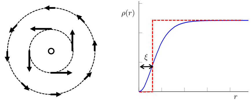
FIGURE IV.4. Gauche : champ de vitesse créé par un vortex, décroissant comme 1/r . Droite : profil de densité au voisinage du cœur du vortex. La taille du cœur est de l'ordre de la longueur de cicatrisation \xi = 1/\sqrt{\tilde{g}\rho} . En pointillé, modélisation par la fonction en escalier donnée en (IV.4).
