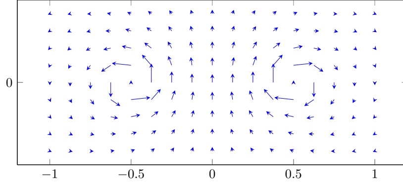
FIGURE IV.7. Champ de vitesses créé par une paire de vortex de charges opposées. Ce champ de vitesses décroît comme 1/r^2 à l'infini et l'énergie cinétique associée est donc bornée quand la taille de l'échantillon tend vers l'infini, contrairement au cas d'un vortex isolé.
