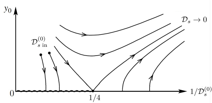
FIGURE IV.9. Trajectoires dans le plan [\mathcal{D}_s^{(0)}, y_0] obtenues par action de la procédure de renormalisation. Figure adaptée de KARDAR (2007).
