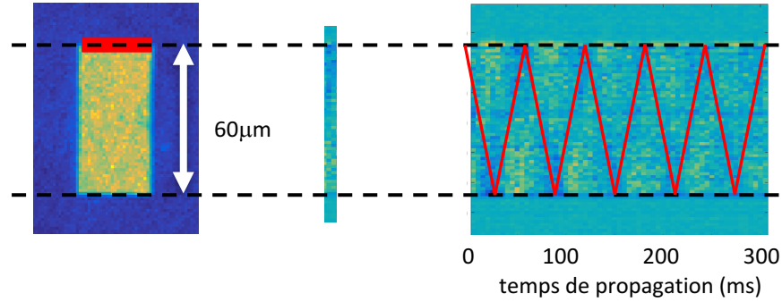
FIGURE III.11. Mise en évidence d'ondes sonores dans un gaz 2D d'atomes de rubidium. Le gaz est confiné dans une boîte rectangulaire et l'onde sonore est générée en modulant brièvement la densité atomique sur un côté de la boîte.
