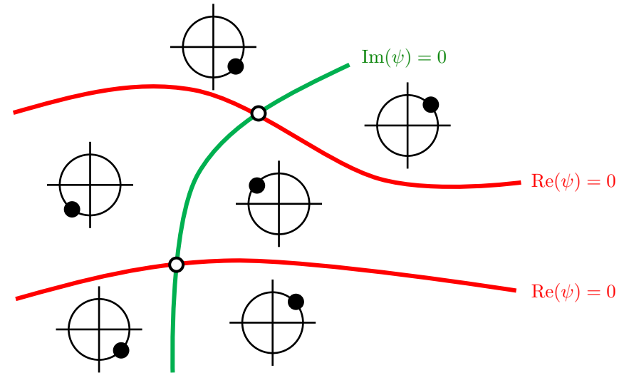
FIGURE IV.2. Lignes sur lesquelles \text{Re}[\psi(\mathbf{r})] = 0 (en rouge) et \text{Im}[\psi(\mathbf{r})] = 0 en vert. Les points d'intersection \mathbf{r}_j sont (généralement) des zéros simples de \psi(\mathbf{r}) et ils correspondent à un enroulement de phase de \pm 2\pi , c'est-à-dire un vortex de charge topologique Q = \pm 1 . On a indiqué dans chaque zone du plan une représentation de la phase de \psi sur le cercle trigonométrique, ce qui permet de déterminer l'enroulement de phase du vortex.
