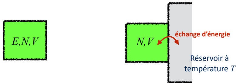
FIGURE VI.1. Gauche, ensemble micro-canonique : système isolé décrit par trois variables extensives : l'énergie E , le nombre de particules N et le volume V . Droite, ensemble canonique : système pouvant échanger de l'énergie avec un réservoir qui impose ainsi sa température T (variable intensive). Le volume et le nombre de particules du système restent fixés.
