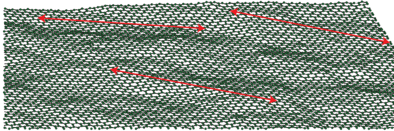
FIGURE I.11. Simulation numérique d'une surface de graphène à 300K, avec N = 8640 atomes, montrant que la surface est plissée sous l'effet des fluctuations thermiques. Les flèches ont une longueur de 8 nm. Figure extraite de FASOLINO, LOS et al. (2007).
