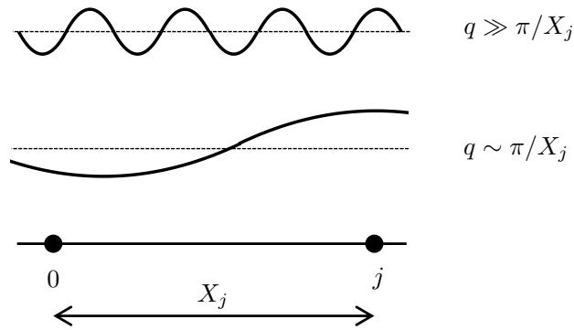
FIGURE I.3. Les deux types de modes susceptibles de contribuer à l'intégrale (I.24), pour une distance X_j donnée entre les deux sites considérés.
