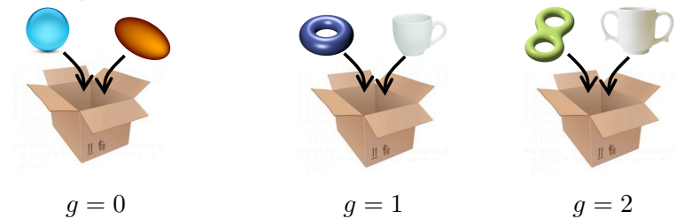
FIGURE 1. Des objets de genre g = 0, 1, 2 .
