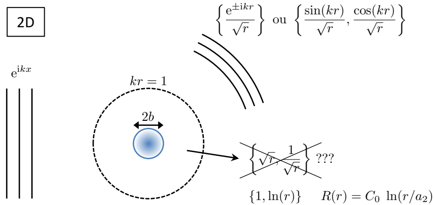
FIGURE II.12. Principe du calcul de l'amplitude de diffusion à 2D par un potentiel ne prenant des valeurs significatives que pour r < b et pour des faibles vecteurs d'onde kb \ll 1 . Pour kr \gg 1 , la superposition de l'onde plane incidente et de l'onde sphérique divergente peut s'écrire après moyenne angulaire comme combinaison linéaire de e^{\pm ikr}/\sqrt{r} . Ces deux fonctions sont les formes asymptotiques des fonctions de Bessel de première et deuxième espèce. Elles se raccordent dans la zone intermédiaire b < r < k^{-1} aux deux fonctions R^{(I)}(r) = \ln(r) et R^{(II)}(r) = 1 . La combinaison linéaire physiquement pertinente, avec notamment la régularité requise en r = 0 , permet de définir la longueur de diffusion a_2 .
