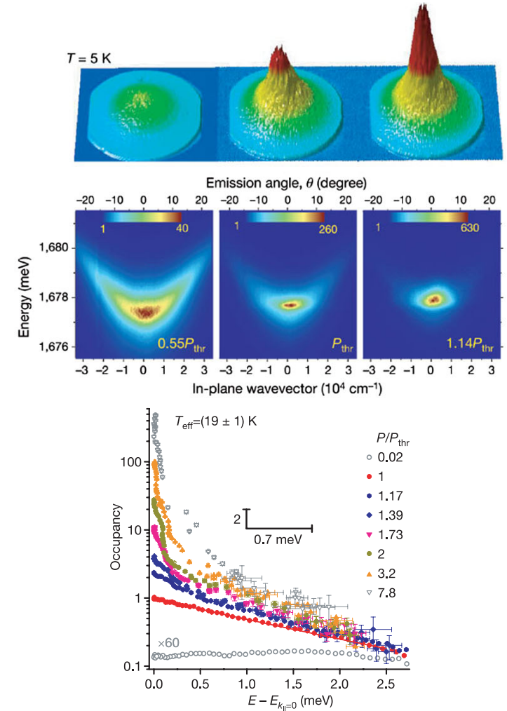
FIGURE V.11. Spectre de la lumière émise par la micro-cavité quand on varie la puissance de pompe. Au dessus d'un certain seuil, la lumière émise est concentrée autour de k_{\perp} = 0 , signalant l'accumulation macroscopique de polaritons au voisinage de ce point. La population des états de grande énergie est saturée. L'expérience est faite à 5 K. Figure extraite de KASPRZAK, RICHARD et al. (2006).
