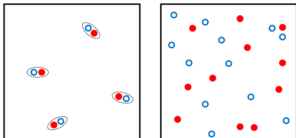
FIGURE 5. Gauche : basse température, défauts topologiques appariés; si on fait une "moyenne à gros grains" de l'état du système, tout se passe comme si les défauts n'étaient pas présents. Droite : haute température, défauts topologiques non appariés; la phase obtenue est radicalement différente de celle attendue à basse température.
