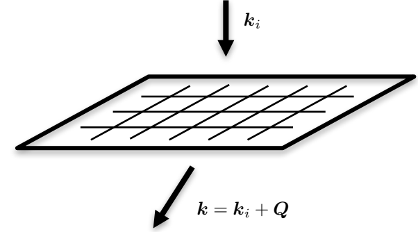
FIGURE I.5. Diffraction de Bragg d'une onde incidente de vecteur d'onde \mathbf{k}_i vers un vecteur d'onde final \mathbf{k} . On a choisi ici \mathbf{k}_i orthogonal au plan des atomes. L'intensité I(\mathbf{k}) révèle un possible ordre ou quasi-ordre cristallin.
