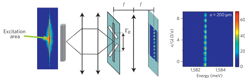
FIGURE V.12. Un fluide de polaritons est créé dans un milieu très allongé. En faisant interférer la lumière issue de deux points séparés d'une distance a , on sonde la cohérence en phase du fluide. La figure de droite obtenue pour a = 200 \mu\text{m} , c'est-à-dire entre les deux extrémités de l'échantillon, montre que la cohérence en phase reste très bonne malgré l'éloignement de ces deux points. Figure extraite de WERTZ, FERRIER et al. (2010).
