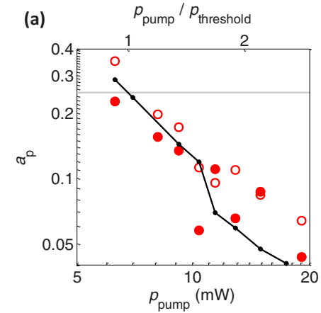
FIGURE V.14. Variation avec la puissance de pompe de l'exposant \alpha_p de la loi algébrique G_1(r) \propto r^{-\alpha_p} . L'exposant mesuré au seuil de la transition est compatible avec la borne supérieure 0.25. Figure extraite de NITSCHKE, KIM et al. (2014).
