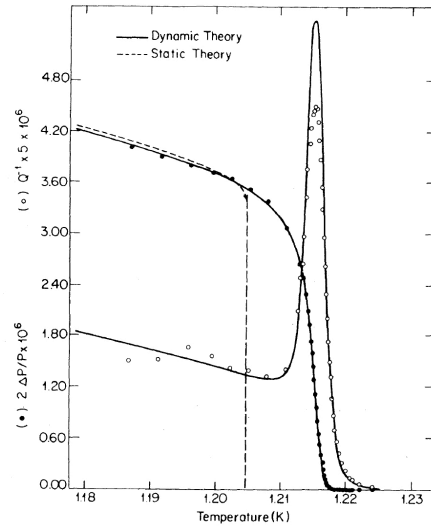
FIGURE IV.11. Ajustement des données expérimentales avec la théorie BKT dynamique de AMBEGAOKAR, HALPERIN et al. (1978). La courbe en pointillé représente la théorie BKT statique que nous avons étudiée dans ce chapitre. Les données en symboles ouverts représente l'excès de dissipation Q^{-1} dû au superfluide (non discuté dans ce cours). Figure extraite de BISHOP & REPPY (1978).
