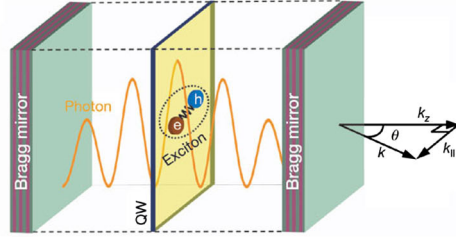
FIGURE V.9. Géométrie utilisée pour les expériences sur les fluides de polaritons de cavité. La lumière est stockée entre deux miroirs plans de grande réflectivité formant une cavité Fabry-Perot résonante. Les excitons sont produits dans un puits quantique. Un polariton est un boson composite, superposition d'un exciton et d'un photon. On sonde les propriétés du fluide de polaritons en analysant les propriétés de la lumière sortant de la cavité. Figure extraite de KASPRZAK, RICHARD et al. (2006).
