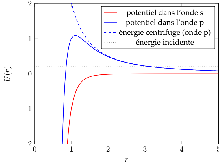
FIGURE II.10. Potentiel radial en -1/r^6 ressenti par une particule dans l'onde s (en rouge, pas de terme centrifuge), et dans une onde partielle de moment cinétique non nul (en bleu, avec un terme centrifuge en +1/r^2 ). Les échelles de longueur et d'énergie sont choisies ici adimensionnées.
