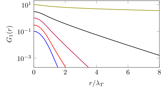
FIGURE II.3. Fonction de corrélation G_1(r) pour un gaz de Bose idéal à deux dimensions. Courbes réalisées pour \mathcal{D} = 0.1, 0.3, 1, 3, 10 .
