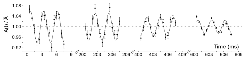
FIGURE VI.8. Oscillation temporelle de l'aire transverse d'un gaz 3D de rubidium confiné dans un piège « cigare ». L'oscillation se fait à une fréquence égale (à la précision de mesure près) au double de la fréquence transverse du piège. Ce mode d'oscillation n'est que très faiblement amorti (facteur de qualité > 2000 ). Figure extraite de CHEVY, BRETIN et al. (2001).
