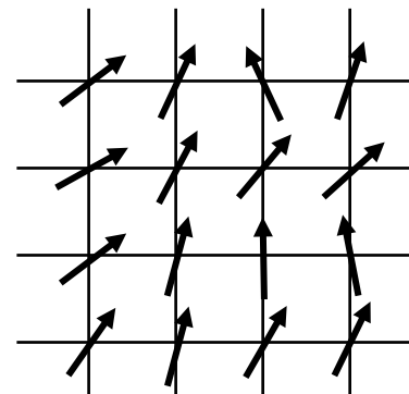
FIGURE III.8. Le modèle xy à deux dimensions, qui peut être considéré comme la version discrétisée du gaz de Bose dont on a gelé les fluctuations de densité.
