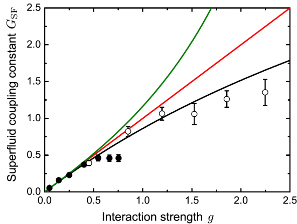
FIGURE VI.7. Paramètre G = m/(\hbar^2 \kappa) , caractérisant le lien entre densité \rho et potentiel chimique \mu à très basse température pour un gaz 2D d'atomes de césium. La théorie de champ classique prédit G = \tilde{g} (ligne droite rouge). La ligne noire continue représente une prédiction basée sur la théorie de Ginzburg–Landau (SACHDEV & DEMLER 2004). Les symboles ouverts ont été obtenus pour un gaz évoluant dans un réseau optique opérant dans un régime où son effet est essentiellement une renormalisation de la masse et de la force des interactions. Figure extraite de HA, HUNG et al. (2013).
