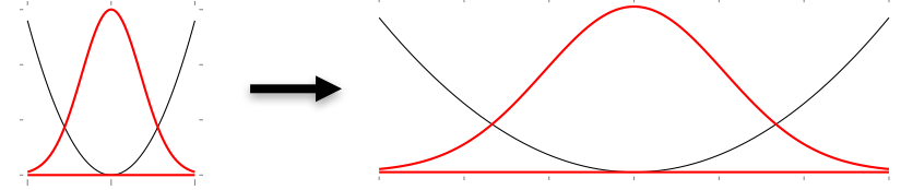
FIGURE II.4. Limite thermodynamique dans un piège : on diminue la pulsation \omega tout en augmentant le nombre d'atomes de manière à garder la densité centrale constante.
