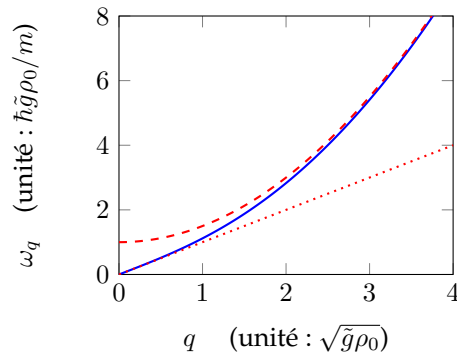
FIGURE III.10. Relation de dispersion de Bogoliubov (III.104). La droite pointillée correspond à l'approximation linéaire (III.106) aux petites valeurs de q déterminant le régime de phonons. La courbe parabolique en tirets correspond aux grandes valeurs de q où l'on retrouve le régime de particule libre (III.108).
