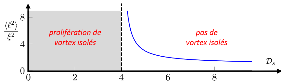
FIGURE IV.8. Variation de l'élongation moyenne d'une paire de vortex en fonction de la densité dans l'espace des phases associée à la fraction superfluide [cf. eq. (IV.28)].
