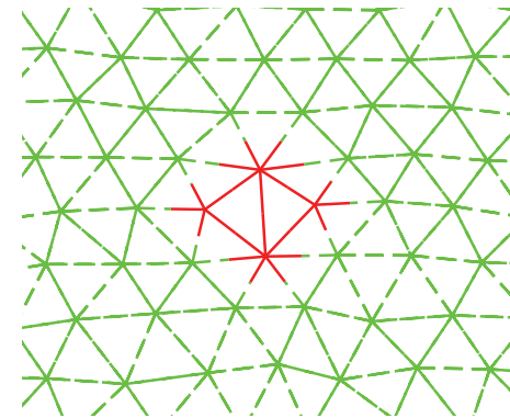
FIGURE I.6. Un défaut local dans une assemblée de particules présentant un quasi-ordre translationnel à longue portée. Ce défaut peut être vu comme une paire de dislocations, avec deux sites A_5 (à cinq voisins) et deux sites A_7 (à sept voisins). Figure extraite de WIERSCHEM & MANOUSAKIS (2011).
