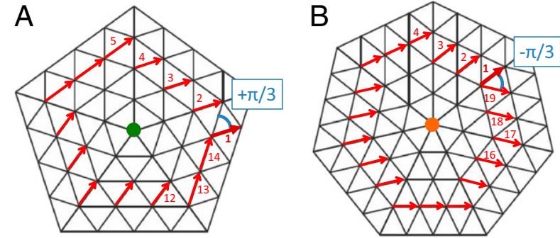
FIGURE I.8. Disclinations correspondant à un défaut de type A_5 ou A_7 . La prolifération de ce type de défaut induit une perte de l'ordre orientationnel. Figure extraite de DEUTSCHLÄNDER, DILLMANN et al. (2015).
