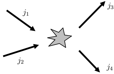
FIGURE III.1. Collision élastique entre deux particules permettant d'assurer l'atteinte de l'équilibre thermique. La conservation de l'énergie impose E_1 + E_2 = E_3 + E_4 .
