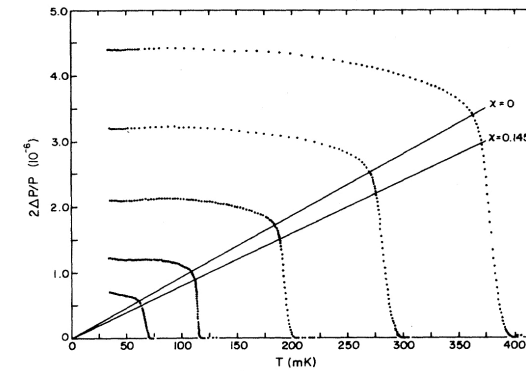
FIGURE IV.12. Mesure de la transition BKT pour différentes quantités d’hélium adsorbées sur le Mylar, montrant le déplacement de la température de transition T_c et le saut de la densité superfluide \rho_s . La loi \Delta\rho_s \propto T prédite par la théorie BKT correspond aux lignes droites en trait plein. Le paramètre phénoménologique \chi appelé obstruction géométrique (geometric hindrance) représente la fraction de superfluide qui n’est pas libre de se déplacer par rapport au Mylar du fait d’imperfections dans l’enroulement de la feuille; sa valeur expérimentale, mesurée indépendamment, est de 0.145. Figure extraite de AGNOLET, MCQUEENEY et al. (1989)
