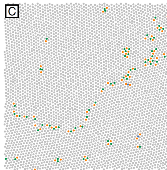
FIGURE I.10. Identification de défauts dans une assemblée d'environ 4000 billes paramagnétiques. Cette figure a été obtenue pour le rapport \Gamma = 98 , après une trempe de pente \dot{\Gamma} = 1/(19 \text{ jours}) . Figure extraite de DEUTSCHLÄNDER, DILLMANN et al. (2015).
