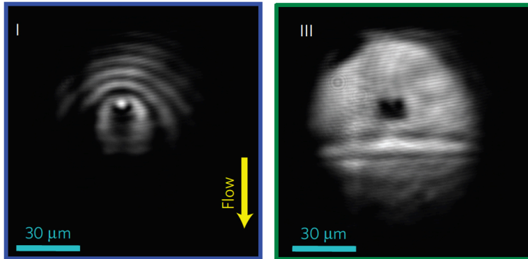
FIGURE V.15. Écoulement d'un fluide de polaritons de vitesse \sim 6 \cdot 10^5 m/s autour d'un obstacle statique. À basse densité (image de gauche), une trainée claire apparaît dans le sillage de l'objet. À haute densité, ce sillage disparaît, indication d'un écoulement superfluide. La vitesse du son pour l'image de droite est de l'ordre de 2 \cdot 10^6 m/s. Figure extraite de AMO, LEFRÈRE et al. (2009).
