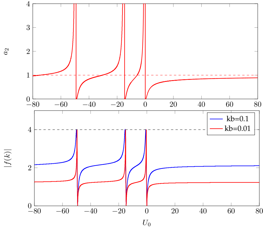
FIGURE II.13. Haut : variation de la longueur de diffusion a_2 (en unité de b ) en fonction de la profondeur du puits U_0 (en unité de \hbar^2/(2m_r b^2) ). Bas : module de l'amplitude de diffusion f(k) pour deux valeurs du vecteur d'onde, kb = 0.1 et kb = 0.01 . Cette amplitude est calculée directement à partir de (II.116) et (II.123) (ou de son équivalent quand la région centrale est classiquement permise). On vérifie numériquement que ce résultat est très proche de l'expression asymptotique (VI.79).
