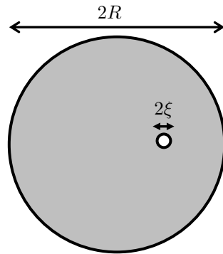
FIGURE IV.5. Un vortex de rayon \approx \xi dans un disque de rayon R .
