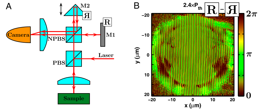
FIGURE V.13. Pour sonder la cohérence en phase d'un fluide de polaritons bi-dimensionnel, on fait interférer la lumière émise avec son image miroir, ce qui permet de reconstruire la fonction de corrélation G_1(\mathbf{r}, -\mathbf{r}) . Figure extraite de ROUMPOS, LOHSE et al. (2012).
