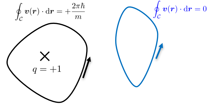
FIGURE III.3. Quantification de la circulation de la vitesse \mathbf{v}(\mathbf{r}) = \frac{\hbar}{m} \nabla \theta associée au champ classique \psi(\mathbf{r}) = \sqrt{\rho(\mathbf{r})} e^{i\theta(\mathbf{r})} . La valeur de la circulation ne peut changer que si le contour \mathcal{C} passe sur un vortex, c'est-à-dire un point où \rho(\mathbf{r}) s'annule.
