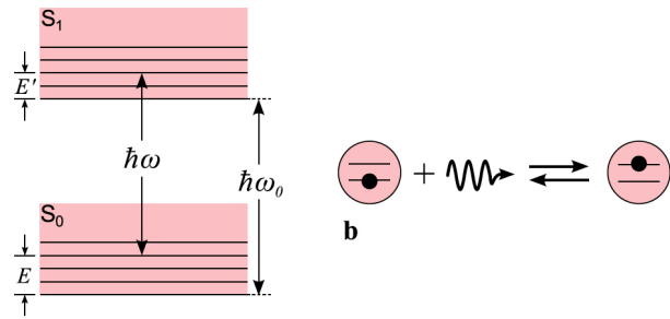
FIGURE II.6. Absorption et émission d'un photon par une molécule de colorant. Figure extraite de KLAERS, SCHMITT et al. (2011).
