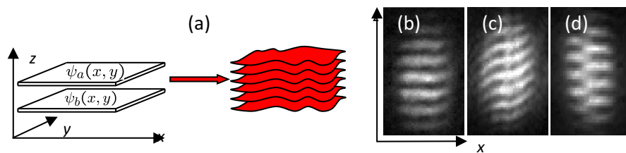
FIGURE V.4. (a) Interférences entre deux plans atomiques indépendants, de même température et de même potentiel chimique. La mesure du contraste de l'interférence observée après expansion selon l'axe z permet d'accéder au module carré de la fonction de corrélation G_1 . (b-c) Figures d'interférence obtenues pour deux températures différentes, en imageant le nuage d'atomes le long de la direction y . (d) Exemple de dislocation de la figure d'interférence révélant la présence d'un vortex dans l'un des deux plans. Figures extraites de HADZIBABIC, KRÜGER et al. (2006).
