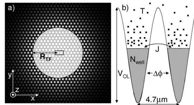
FIGURE III.9. Réseau triangulaire de micro-condensats piégés aux nœuds d'un réseau optique, avec un couplage tunnel entre proches voisins. Chaque site contient environ 7000 atomes, ce qui assure que la phase d'un micro-condensat est bien définie. Cette expérience constitue une implémentation pratique du modèle xy . Figure extraite de SCHWEIKHARD, TUNG et al. (2007).
