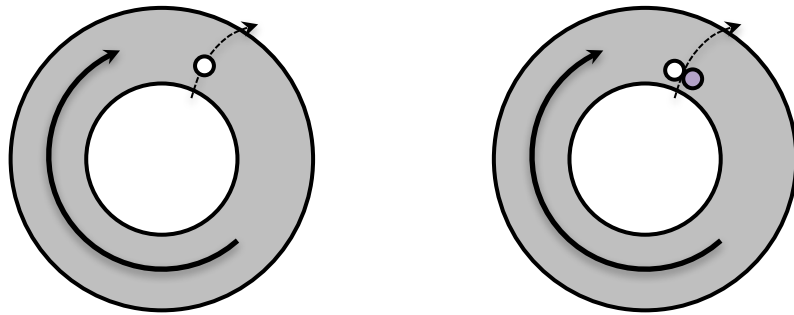
FIGURE IV.6. Gauche : quand un anneau de fluide bi-dimensionnel est traversé par un vortex isolé, le courant (quantifié) dans cet anneau est modifié. On ne peut donc pas avoir de courant permanent – condition nécessaire de superfluidité – dès que les vortex isolés ont une probabilité significative de se trouver au sein du fluide. Droite : la traversée d'une paire liée de deux vortex de charges opposées n'a en revanche pas d'effet sur le courant permanent.
