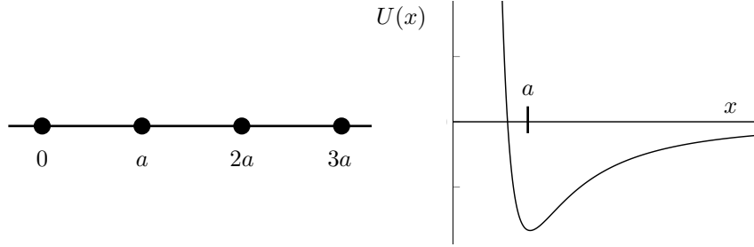
FIGURE I.1. Chaîne uni-dimensionnelle d'atomes avec des interactions entre proches voisins décrites par le potentiel U(x) . Ce potentiel a un minimum en x = a , ce qui a pour effet de former un cristal, au moins pour un gaz de particules à température nulle décrites par la physique classique (pas de fluctuations thermiques, ni quantiques).
