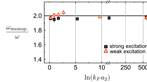
FIGURE VI.9. Fréquence du mode monopolaire d'un gaz 2D de fermions ( ^{40}\text{K} ) au voisinage d'une résonance de Feshbach. La longueur de diffusion a_2 est mesurée ici en unités du vecteur d'onde de Fermi k_F ( E_F = \hbar^2 k_F^2 / 2m \approx 5 à 8 \text{ kHz} \times \hbar ). On trouve que la fréquence du mode monopolaire reste très proche de la valeur prédite dans le cadre de l'invariance d'échelle, même quand la longueur de diffusion a_2 devient grande. Figure extraite de VOGT, FELD et al. (2012).
