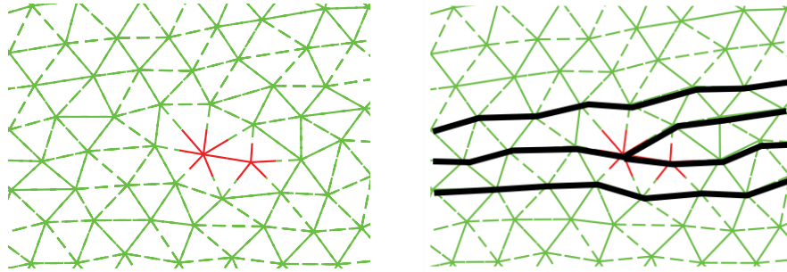
FIGURE I.7. Dislocation isolée composée d'un site A_5 et d'un site A_7 , ce qui revient à insérer une demi-ligne supplémentaire d'atomes. Figure extraite de WIERSCHEM & MANOUSAKIS (2011).
