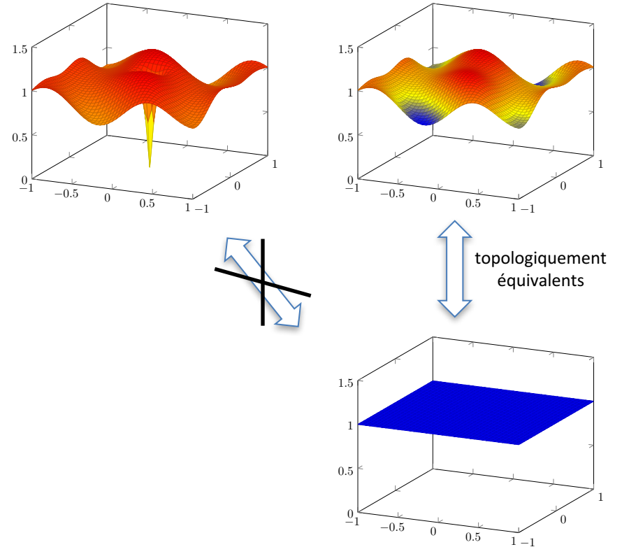
FIGURE 4. Gauche : amplitude du champ \psi(\mathbf{r}) contenant un vortex. Ce "défaut" est protégé topologiquement du fait de l'enroulement de phase de \pm 2\pi autour de lui. Droite : amplitude d'un champ \psi(\mathbf{r}) ne présentant que des oscillations douces de \rho(\mathbf{r}) et \theta(\mathbf{r}) , avec \rho(\mathbf{r}) ne s'annulant nulle part. Ce champ peut être déformé continûment en un champ uniforme, correspondant à l'état attendu à température nulle.
