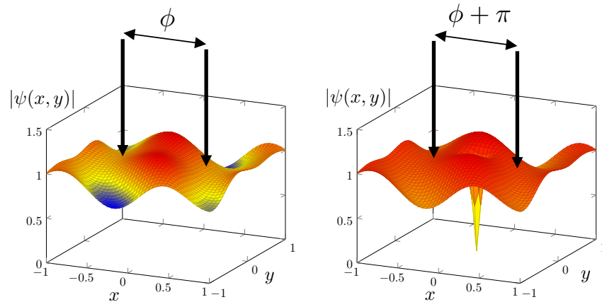
FIGURE IV.1. Vortex isolés et cohérence de phase : si un vortex isolé vient s'intercaler entre deux points, la phase relative entre ces deux points passe de la valeur \phi à \phi + \pi . Par conséquent, dans un fluide où les vortex isolés peuvent être répartis de manière aléatoire, la cohérence de phase ne peut pas excéder une longueur de l'ordre de la distance moyenne entre vortex.
