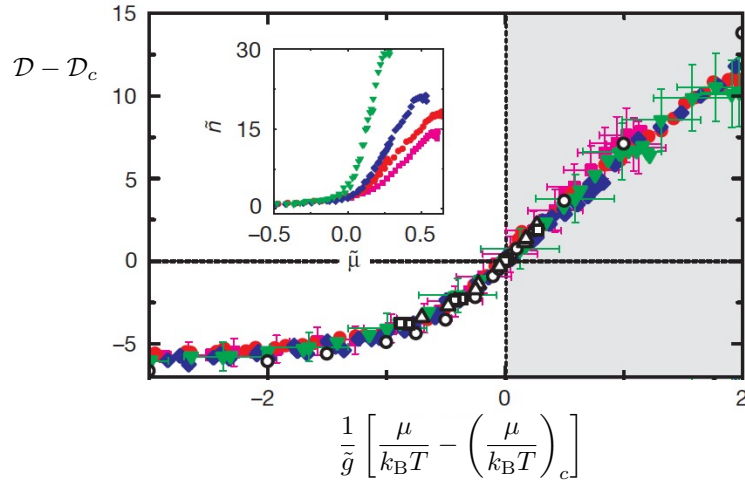
FIGURE VI.6. Ecart entre la densité dans l'espace des phases \mathcal{D} et sa valeur critique \mathcal{D}_c , en fonction du paramètre "universel" défini en (VI.63). Le paramètre \tilde{g} vaut 0.05 (triangles verts), 0.13 (losanges bleus), 0.19 (cercles rouges) and 0.26 (carrés magenta). L'insert représente la variation de \mathcal{D} en fonction de \mu/k_B T . Ces mesures sont faites sur un gaz de césium au voisinage d'une résonance de Feshbach. Figure extraite de HUNG, ZHANG et al. (2011).
