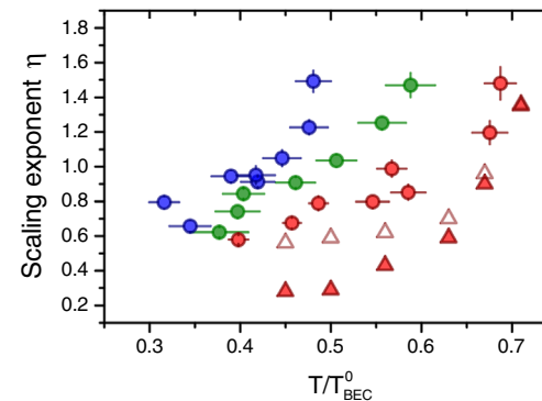
FIGURE V.6. Cercles : exposant \eta obtenu par ajustement des données expérimentales avec une loi algébrique \alpha r^{-\eta} , pour les paramètres d'interaction \tilde{g} = 0.60 (rouge), 1.07 (vert) et 2.76 (bleu). Triangles pleins : résultats d'une simulation Monte Carlo quantique pour \tilde{g} = 0.60 . Triangles évidés : idem avec en plus la prise en compte de la résolution finie du système d'imagerie. Figure extraite de MURTHY, BOETTCHER et al. (2015).
