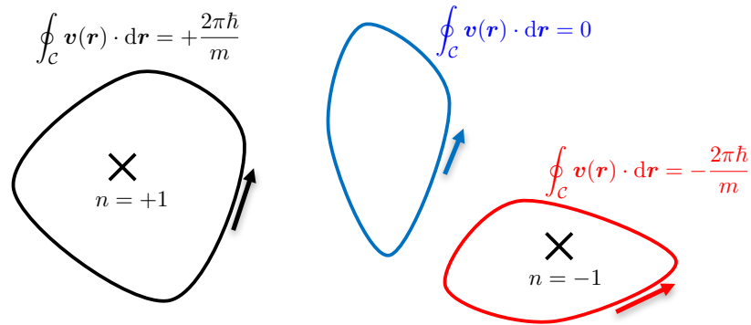
FIGURE 3. Circulation du champ de vitesse sur un contour fermé C dans un gaz bi-dimensionnel de bosons. Cette circulation est non nulle si le contour englobe un vortex. La valeur est alors quantifiée [équation (4)] avec l'entier n qui donne la charge du vortex (ou la somme des charges si plusieurs vortex se trouvent à l'intérieur du contour).
