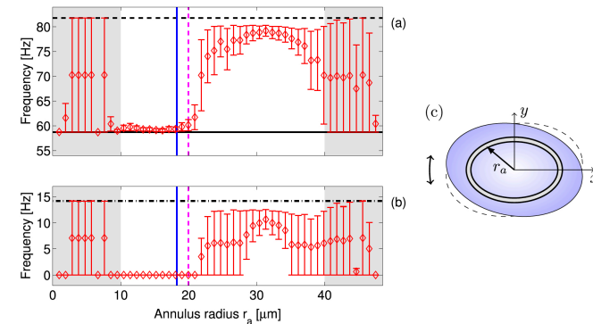
FIGURE V.8. Mode « ciseaux » observé sur un gaz 2D de rubidium en utilisant une analyse de la moyenne locale de la quantité xy , moyenne prise sur un anneau fin. Selon la position de l'anneau, on sonde (i) la région centrale superfluide, avec une seule fréquence d'oscillation ; (ii) la région périphérique normale, avec deux fréquences d'oscillation non nulles. Figure extraite de DE ROSSI, DUBESSY et al. (2016).
