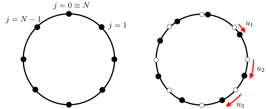
FIGURE I.2. Gauche : chaîne ordonnée de N atomes avec des conditions aux limites périodiques, conduisant à identifier l'atome j = 0 et l'atome j = N . Droite : définition des déplacements u_j par rapport aux positions d'équilibre. On suppose que |u_{j+1} - u_j| \ll a mais pas nécessairement que |u_j| \ll a .
