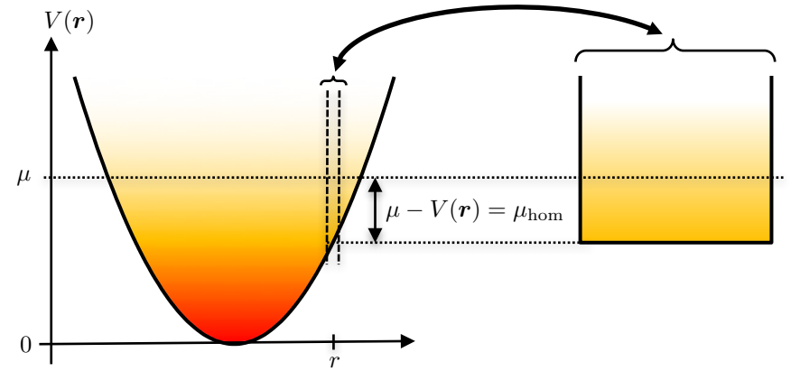
FIGURE V.1. Principe de l'approximation de densité locale : l'état d'équilibre du gaz au point \mathbf{r} dans un piège V(\mathbf{r}) est similaire à celui d'un gaz homogène de même température et de potentiel chimique \mu_{\text{hom.}} = \mu - V(\mathbf{r}) .
