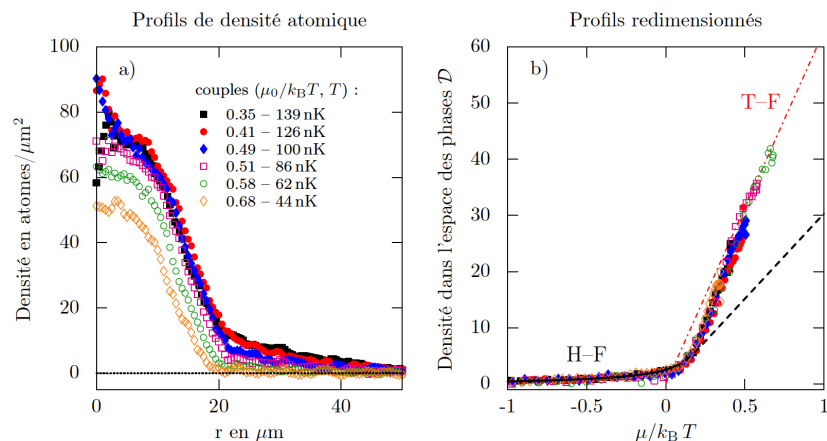
FIGURE VI.4. Vérification de l'invariance d'échelle pour un gaz 2D de ^{87}\text{Rb} en interaction relativement faible, \tilde{g} = 0.1 . Les profils de densité \rho(r) mesurés dans un potentiel V(r) se regroupent sur une courbe unique si on trace la densité dans l'espace des phases \mathcal{D}(r) = \rho(r)\lambda_T^2 en fonction de \mu_{\text{loc}}(r)/k_B T . Les deux régimes Hartree-Fock (HF) et Thomas-Fermi (TF) correspondent respectivement au cas faiblement et fortement dégénérés. Figure extraite de la thèse de Tarik YEFSAH (2011).
