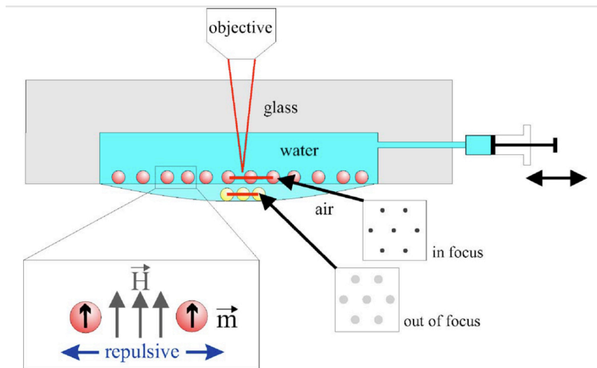
FIGURE I.9. Montage expérimental utilisé dans les expériences de Constance. Une goutte d'eau de diamètre 8mm est suspendue par capillarité. Des billes de polystyrène dopées par des nanoparticules d'oxyde de fer s'accumulent sur le plan inférieur, à l'interface eau-air. Un champ magnétique vertical induit un moment magnétique dans les billes, ce qui crée une interaction répulsive entre billes. Figure extraite de KEIM, MARET et al. (2007).
