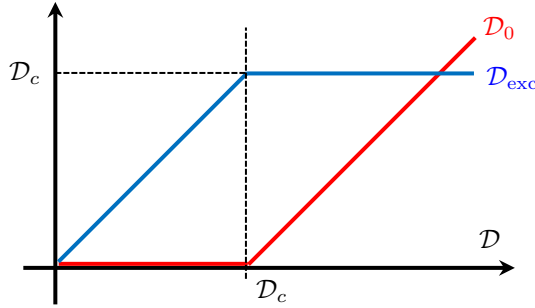
FIGURE II.1. Cas 3D : densités dans l'espace des phases associées respectivement à l'état fondamental ( \mathcal{D}_0 ) et à l'ensemble des états excités \mathcal{D}_{\text{exc}} , en fonction de la densité totale dans l'espace des phases \mathcal{D} . On a posé \mathcal{D}_c \equiv \mathcal{D}_{\text{exc}}^{\text{max}} = 2.612 .
