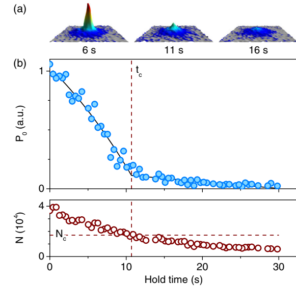
FIGURE V.2. Méthode utilisée par FLETCHER, ROBERT DE SAINT VINCENT et al. (2015) pour mesurer le point critique de la transition BKT dans un piège harmonique 2D ( \nu_{xy} = 38 Hz). Le gaz est \approx dans le régime 2D car la température T \sim 150 nK est telle que k_B T < \hbar \nu_z , avec \nu_z = 4.1 kHz.
