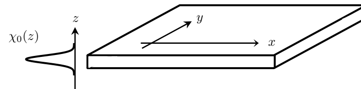
FIGURE III.4. Fonction d'onde \chi_0(z) correspondant au gel du mouvement dans la direction z .
