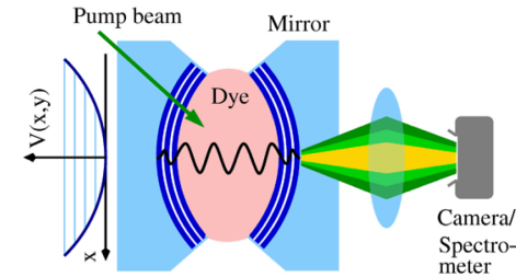
FIGURE II.5. Cavité Fabry-Perot remplie de colorant et pompée latéralement par un laser. Pour un taux de pompage suffisamment élevé, la condensation de Bose–Einstein de photons se produit dans le mode longitudinal N = 7 et dans le mode transverse fondamental. Figure extraite de KLAERS, SCHMITT et al. (2011).
