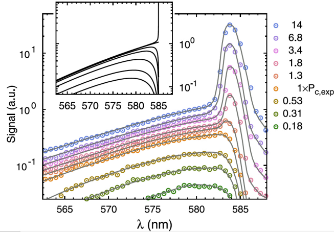
FIGURE II.7. Spectre de la lumière émise pour différentes puissances de pompe. Les lignes continues sont des ajustements par des distributions de Bose–Einstein associées à l'énergie (II.71) et de fugacité non nulle. Pour une puissance de pompe supérieure à un certain seuil, une accumulation macroscopique de photons se produit dans le mode fondamental de la cavité. Figure extraite de KLAERS, SCHMITT et al. (2011).
