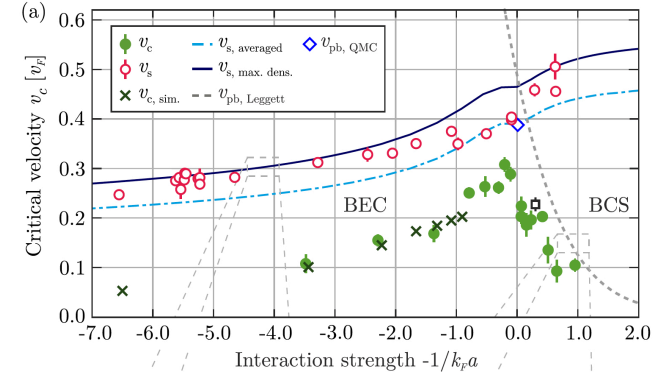
FIGURE V.7. Comportement superfluide d'un gaz de fermions ( {}^6\text{Li} ). Haut : variation de la densité centrale (i.e. chauffage) induit par une impureté bougeant à vitesse v dans la partie superfluide ou la partie normale du gaz. Bas : vitesse critique (points verts) et vitesse du son (points rouges) en unité de la vitesse de Fermi v_F dans la zone de transition entre le condensat de molécules {}^6\text{Li}_2 et le régime de paires de Cooper. Figure extraite de WEIMER, MORGENER et al. (2015).
