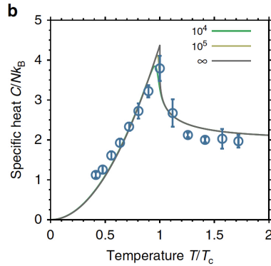
FIGURE II.9. Chaleur spécifique (par photon) mesurée en fonction de la température réduite T/T_c , montrant la singularité caractéristique de la transition de Bose–Einstein. Dans le régime de haute température, la chaleur spécifique atteint la limite classique de 2k_B par photon. Les lignes continues donnent la prédiction pour un gaz de Bose idéal pour trois nombres de particules différents. Figure extraite de DAMM, SCHMITT et al. (2016).
