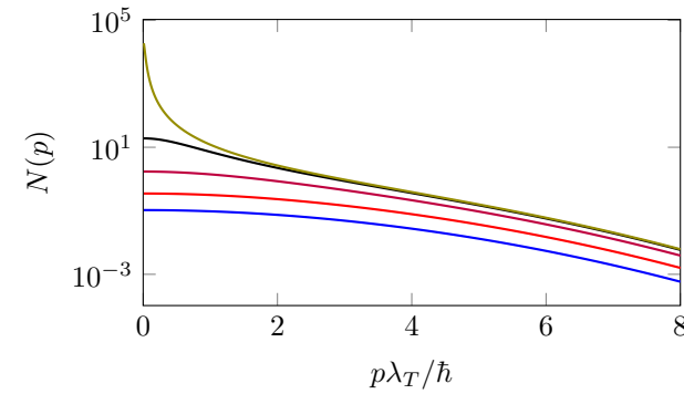
FIGURE II.2. Distributions en impulsion pour \mathcal{D} = 0.1, 0.3, 1, 3, 10 .
