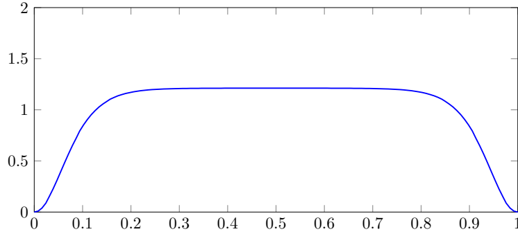
FIGURE III.5. La longueur de cicatrization est la distance caractéristique nécessaire pour que la densité reprenne sa valeur moyenne, quand on impose à la fonction d'onde de s'annuler en un point donné (ici les deux extrémités du segment).
