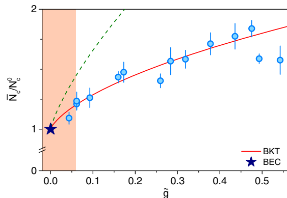
FIGURE V.3. Nombre critique d'atomes pour la transition BKT, ramené au nombre critique d'atomes pour la condensation du gaz parfait, en fonction du paramètre d'interaction \tilde{g} . Dans la zone colorée, la densité dans l'espace des phases au point critique \mathcal{D} = \ln(380/\tilde{g}) devient grande. De ce fait, la longueur de cohérence du gaz \ell \sim \lambda_T e^{D/2} (chapitre 2) est elle aussi très grande avant même d'atteindre le point critique, ce qui rend la détermination du point critique imprécise [figure extraite de FLETCHER, ROBERT DE SAINT VINCENT et al. (2015)].
