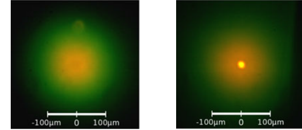
FIGURE II.8. Répartition spatiale de la lumière émise par la cavité, en dessous (gauche) et au-dessus (droite) de la puissance seuil. On notera que les longueurs d'onde les plus courtes (vertes) sont émises sur les bords, confirmant la présence du potentiel harmonique effectif m_{\text{ph}} \Omega^2 r^2 / 2 . Figure extraite de KLAERS, SCHMITT et al. (2011).
