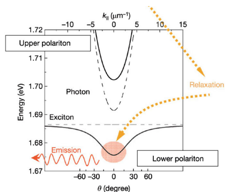
FIGURE V.10. Relation de dispersion ( \mathbf{k} , \hbar\omega_{\text{ex}} ) pour le mouvement d'un polariton dans le plan xy , résultant de l'hybridation entre la relation de dispersion d'un exciton, quasiment plate à cette échelle, et celle d'un photon, qui acquiert une masse effective (très faible) du fait de son confinement dans la cavité Fabry-Perot. Figure extraite de KASPRZAK, RICHARD et al. (2006).
