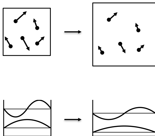
FIGURE VI.3. Dilatation des longueurs par un facteur \lambda dans le cas classique (en haut) et quantique (en bas).
