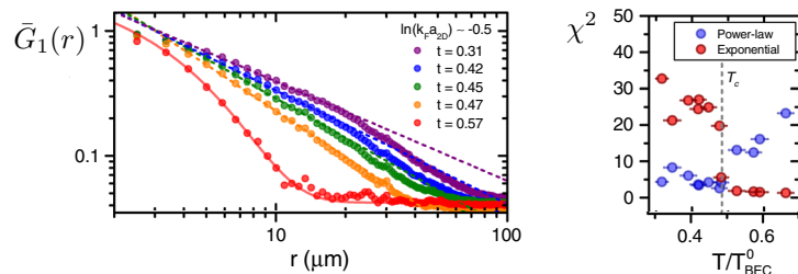
FIGURE V.5. Fonction \bar{G}_1(r) obtenue par transformée de Fourier de la distribution en impulsion, pour un gaz de molécules bosoniques {}^6\text{Li}_2 , avec un paramètre d'interaction \tilde{g} \approx 2.76 . Les températures sont repérées par rapport à la température de condensation d'un gaz parfait dans ce piège : t = T/T_{c,\text{ideal}} avec T_{c,\text{ideal}} = 140 \text{ nK} . A droite : coefficient \chi^2 de l'ajustement par une loi algébrique ( \alpha r^{-\eta} ) ou exponentielle ( \alpha e^{-\eta r} ). Figures extraites de MURTHY, BOETTCHER et al. (2015).
