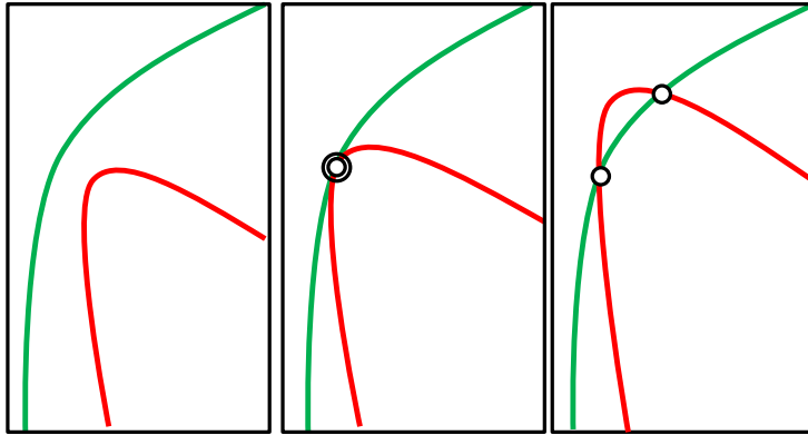
FIGURE IV.3. Emergence d'une paire de vortex du fait de fluctuations thermiques dans le gaz. Sous l'effet d'une fluctuation, la ligne correspondant à \text{Re}[\psi(\mathbf{r})] = 0 (en rouge), initialement disjointe de la ligne \text{Im}[\psi(\mathbf{r})] = 0 (en vert) [dessin de gauche], vient la croiser pour former un zéro double [dessin central], puis en deux zéros simples d'enroulements opposés [dessin de droite]. On obtient alors une paire de vortex de charge Q_1 = +1 et Q_2 = -1 . Le processus inverse est également possible, conduisant à l'annihilation de la paire de vortex.
