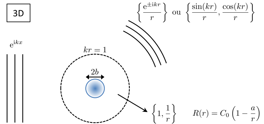
FIGURE II.11. Principe du calcul de l'amplitude de diffusion à 3D par un potentiel ne prenant des valeurs significatives que pour r < b et pour des faibles vecteurs d'onde kb \ll 1 . Pour kr \gg 1 , la superposition de l'onde plane incidente et de l'onde sphérique divergente peut s'écrire après moyenne angulaire comme combinaison linéaire de e^{\pm ikr}/r . Ces deux fonctions de base se raccordent dans la zone intermédiaire b < r < k^{-1} aux deux fonctions R^{(I)}(r) = 1 et R^{(II)}(r) = 1/r . La combinaison linéaire physiquement pertinente, avec notamment la régularité requise en r = 0 , permet de définir la longueur de diffusion a .
