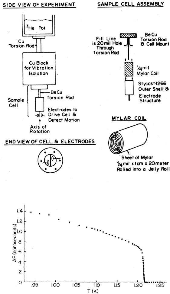
FIGURE IV.10. Haut : schéma expérimental utilisé par BISHOP & REPPY (1978). Une feuille de Mylar de surface \sim 0.4 \text{ m}^2 est recouverte d'un film d'hélium liquide. L'épaisseur de ce film est de l'ordre de quelques couches atomiques seulement. La feuille de Mylar est montée sur un pendule de torsion pour mesurer le moment d'inertie de l'ensemble Mylar+film d'hélium. Bas : Exemple de résultat pour la période du pendule de torsion en fonction de la température du système. La transition superfluide se manifeste par une réduction soudaine du moment d'inertie. Figures extraites de BISHOP & REPPY (1978) et BISHOP & REPPY (1980).
