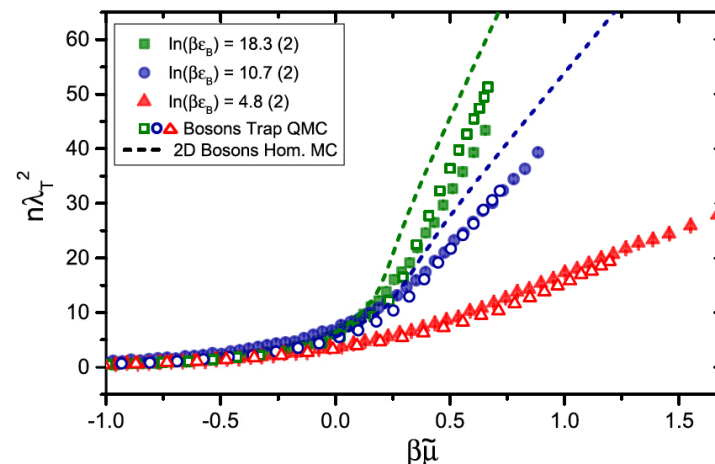
FIGURE VI.5. Symboles fermés : équations d'état mesurées pour un gaz de molécules ^6\text{Li}_2 avec un paramètre d'interaction \tilde{g} = 0.60 (carrés), 1.07 (cercles), 2.75 (triangles). Les lignes pointillées donnent la prédiction obtenue par simulation de champ classique (PROKOF'EV & SVISTUNOV 2002). Les symboles ouverts donnent le résultat d'une simulation de Monte Carlo quantique. Figure extraite de BOETTCHER, BAYHA et al. (2016).
