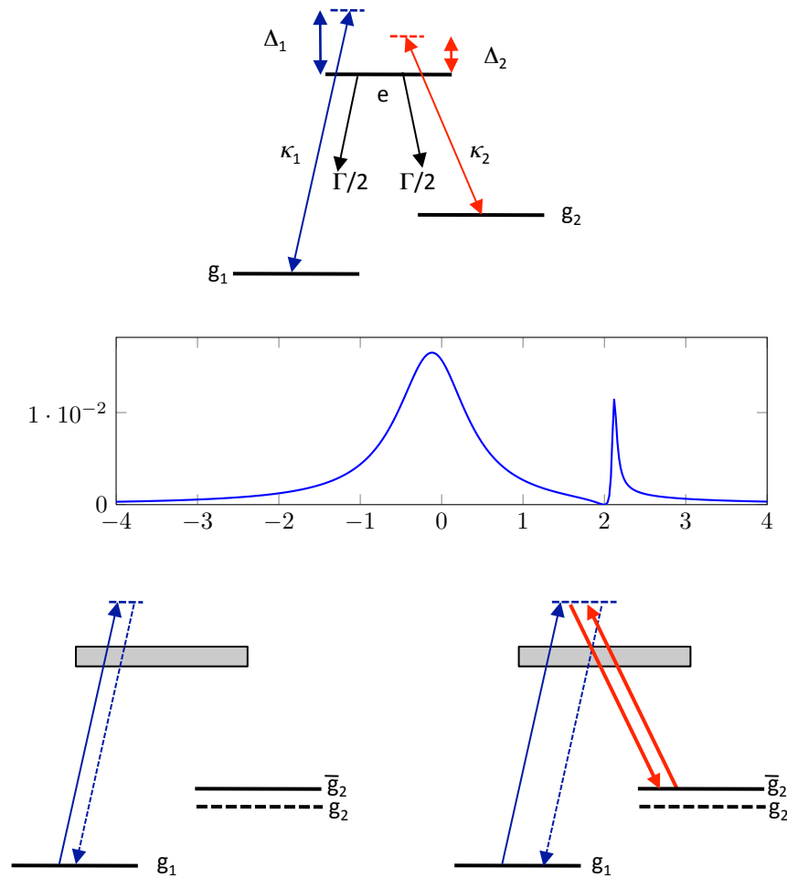
FIGURE V.19. Haut : système modèle en \Lambda . Milieu : Variation de la population excitée P_e avec le désaccord \Delta_1 , mesuré en unité de \Gamma . Les autres paramètres sont (en unités de \Gamma ) : \kappa_1 = 0.1 , \kappa_2 = 1 , \Delta_2 = 2 . (Bas) : Les deux processus de diffusion pour un photon du laser 1, conduisant au profil de Fano de la figure du milieu.
