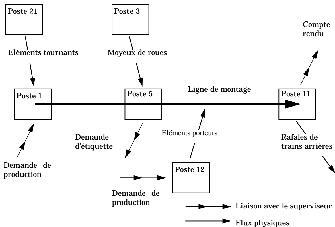
Fig. 2 : structure schématique de la ligne de montage
