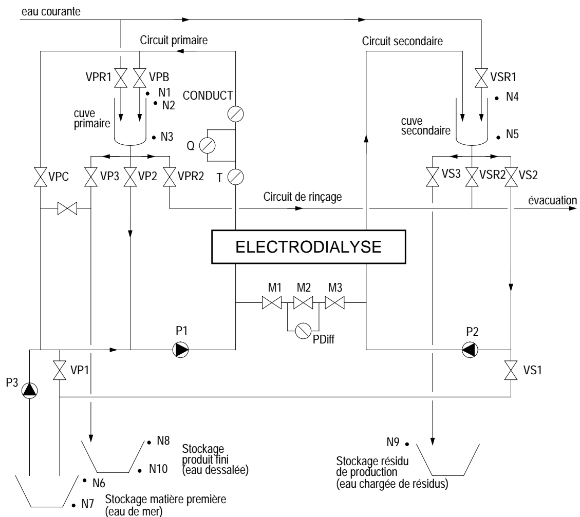
Fig. 1 : processus de SEDEM-91
