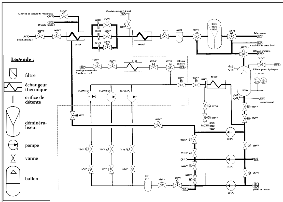
Fig. 3 : schéma simplifié du RCV
