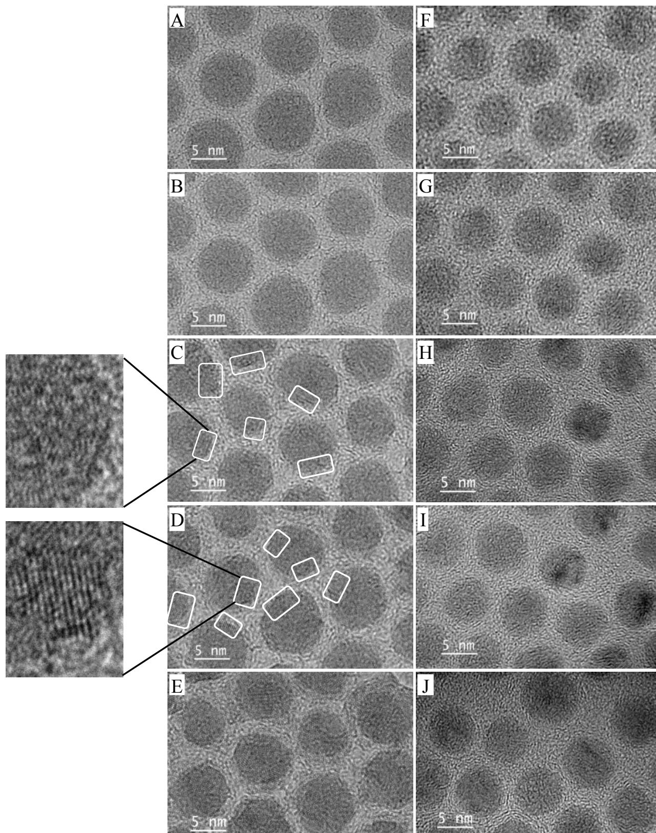
Figure 2. HRTEM images of Co polycrystals under electron beam irradiation for: (A) 0 min, (B) 1.5 min, (C) 6 min, (D) 10 min, (E) 16 min; and of hcp-Co single-crystals for (F) 0 min, (G) 5 min, (H) 7 min, (I) 10 min and (J) 16 min.
