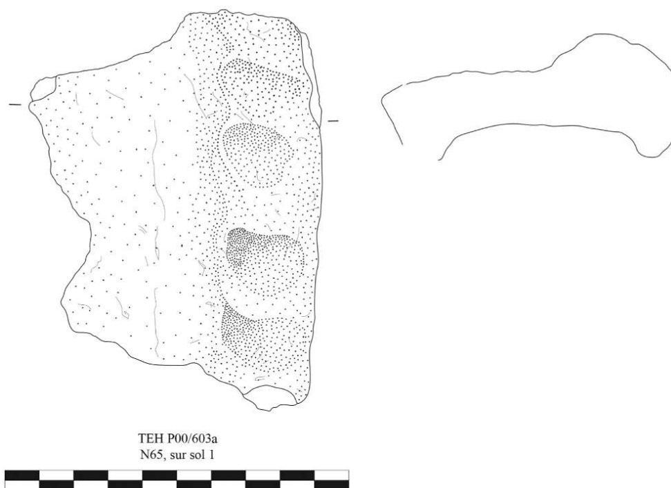
Fig. 7. Dessin d'un fragment de four domestique – secteur nord, phase VA. Inv. TEH P00/603A (A. Banaszak/Mission franco-égyptienne de Tell el-Herr).
