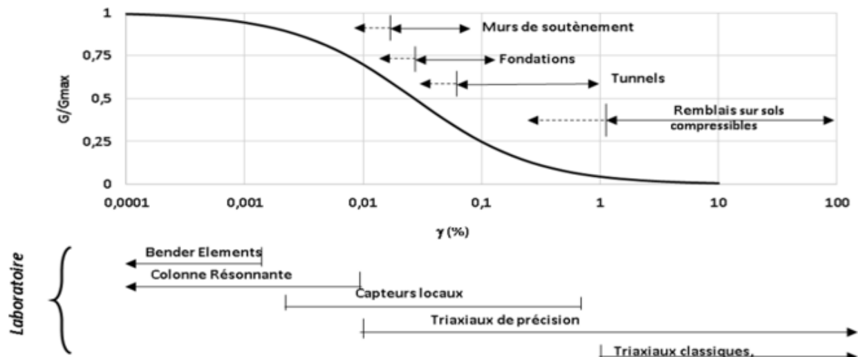
Figure 3. Courbe de réduction du rapport G/G_{max} en fonction de la distorsion pour les différentes plages de déformation propres aux ouvrages et aux essais de laboratoires (d'après Reiffsteck, 2002)
