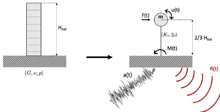
Figure 1. Principe du bâtiment régulier à étages identiques (à gauche) modélisé en oscillateur ancré dans le sol, avec une masse concentrée m à la hauteur H=2/3.H_{\text{bâtiment}} . La raideur de l'ouvrage est K_1 et son amortissement est \xi_0 (Rodet, 2021). Les oscillations du bâtiment sous l'action du signal entrant caractérisé par une accélération a(t) , génèrent une émission de signal vers le sol. M(t) est le moment au niveau de la fondation, F(t) , l'effort horizontal et u(t) le déplacement de la masse m . Le sol est caractérisé par ses paramètres élastiques G , le module de cisaillement et \nu , le coefficient de Poisson ainsi que par son poids volumique \rho ( \text{kg.m}^{-3} ).
