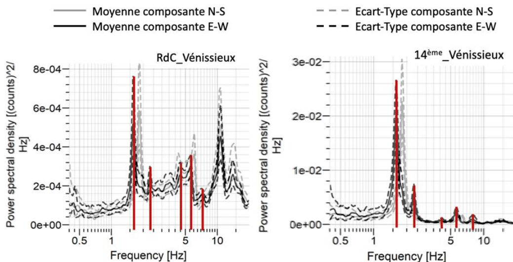
Figure 5. Spectres illustrant la réponse spectrale de la tour HLM de Vénissieux. Ces spectres ont été obtenus à partir de mesures de bruit de fond conventionnelles (Bard et al., 2008) réalisées à l'aide d'un capteur trois composantes Lennartz. Le traitement des données a été effectué avec le logiciel libre GEOPSY (Wathelet et al., 2020).
