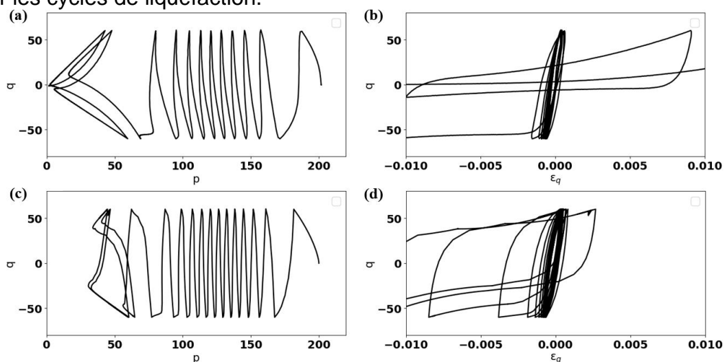
Figure 4. Test cyclique non-drainé contrôlé en contrainte sur du sable fin de Karlsruhe de densité medium: (a) et (b) données par Wichtmann et Triantafyllidis (2016a), (c) et (d) modélisations
