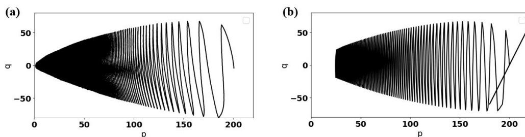
Figure 5. Test cyclique non-drainé contrôlé en déformation sur du sable fin de Karlsruhe de densité médium: (a) données par Wichtmann et Triantafyllidis (2016a), (b) modélisation
