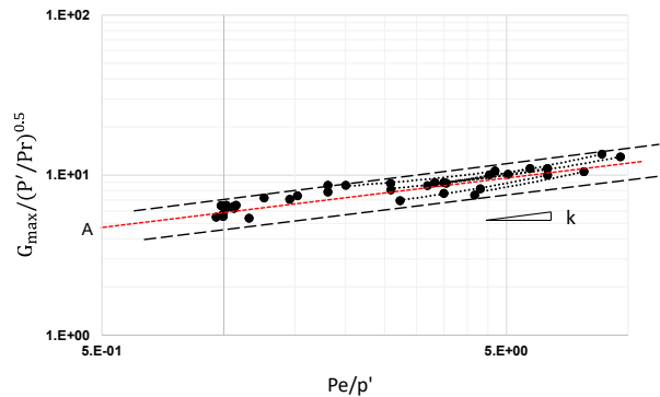
Figure 6 : Normalisation en fonction du taux de surconsolidation R = Pe/p'
