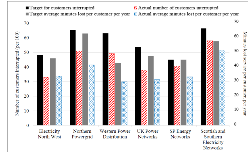
CI & CML (UK, 2016-17)
