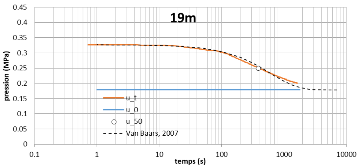
Figure 8 Courbes de dissipation et évaluation de t_{50} pour l'essai à 19 m
