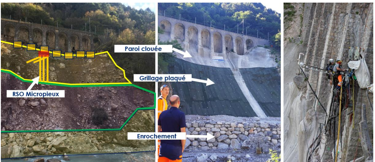
Figure 3. Chantier du mur à arcatures de FONTAN (Avant, après et travaux sur cordes)
