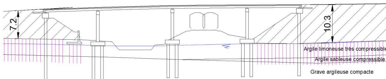
Figure 1: Profil en long schématique du projet
