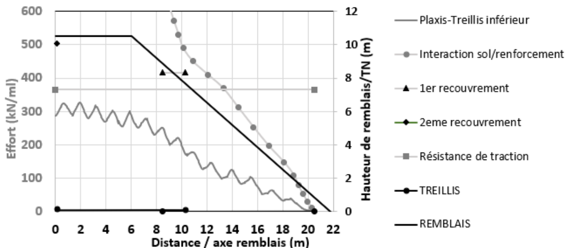
Figure 8: Vérification des efforts dans les treillis – nappe inférieure
