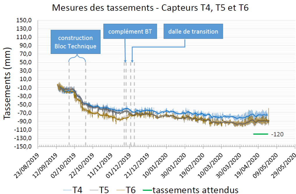
Figure 4: Tassements mesurés
