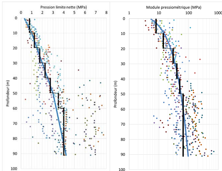
Figure 5 : Résultats des essais pressiométriques
