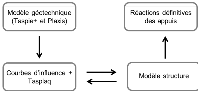
Figure 3 : Principe d'évaluation des raideurs des fondations et procédure d'ISS
