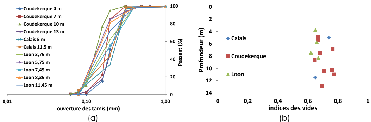
Figure 1. Analyse granulométrique des sables rencontrées sur les trois sites (a) et indices des vides (b)
