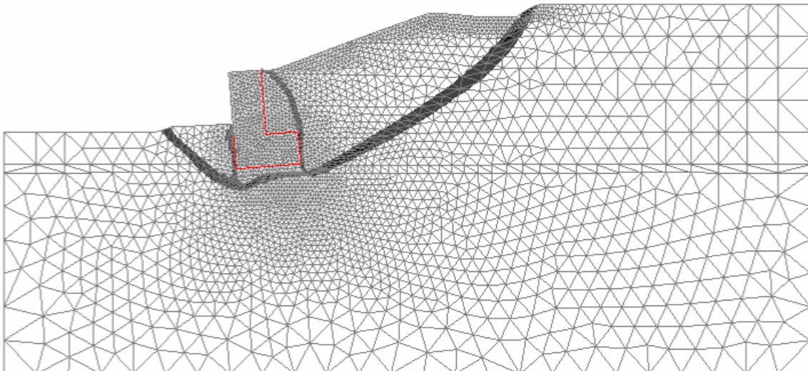
Figure 3. Isosurfaces des déformations plastiques - cas du massif constitué de sable et de marne
