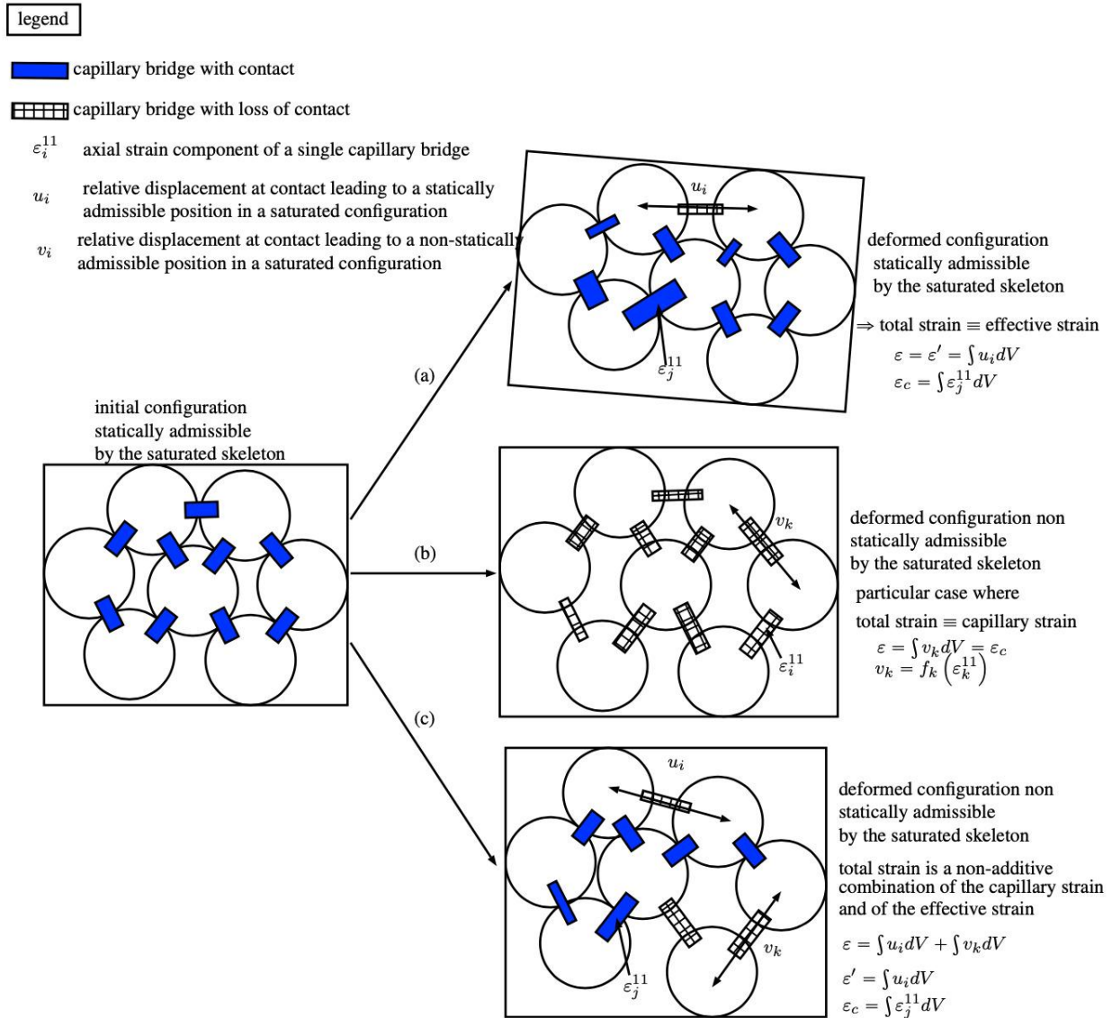
Figure 1. Diagramme de décomposition des déformations dans un milieu granulaire non saturé. Les grains et ponts capillaires sont représentés de manière schématique par des cercles et des rectangles. Le signe intégral indique une opération de sommation sans définition mathématique.
