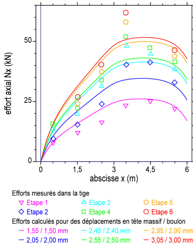
Figure 3. Simulation du chargement d'un boulon radial à ancrage réparti (clou) Effort axial en fonction de l'abscisse ( x , N_x )
