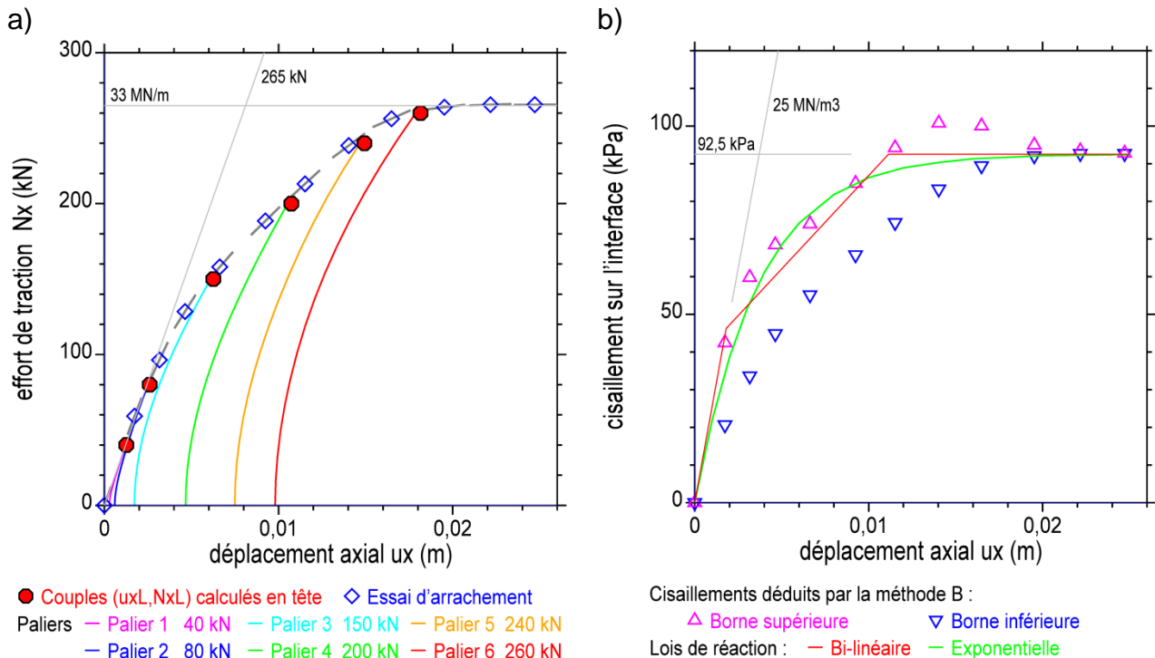
Figure 1. Simulation d'un essai d'arrachement d'un boulon à ancrage réparti (clou) : a) Courbe d'arrachement ( u_{xL}, N_{xL} ) et courbes ( u_x, N_x ) le long du boulon b) Contraintes de cisaillement sur l'interface en fonction du déplacement axial ( u_x, \tau_x )
