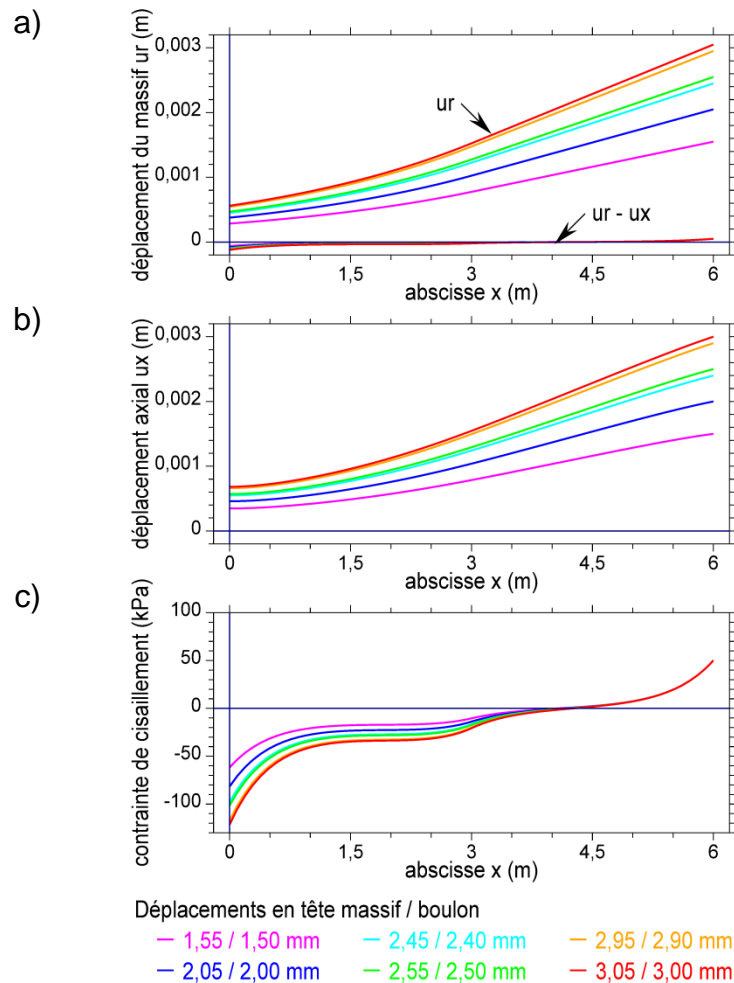
Figure 4. Simulation du chargement d'un boulon radial à ancrage réparti (clou)
