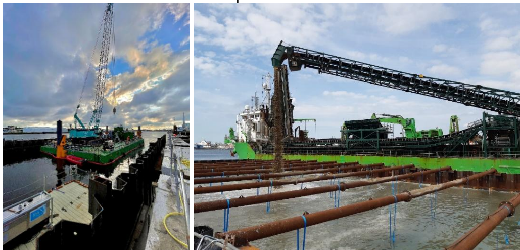
Figure 7. Réalisation du batardeau (Mise en œuvre / Remplissage)
