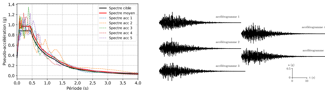
Figure 6. Comparaison du spectre moyen à 5% des accélérogrammes calculés et spectre cible
