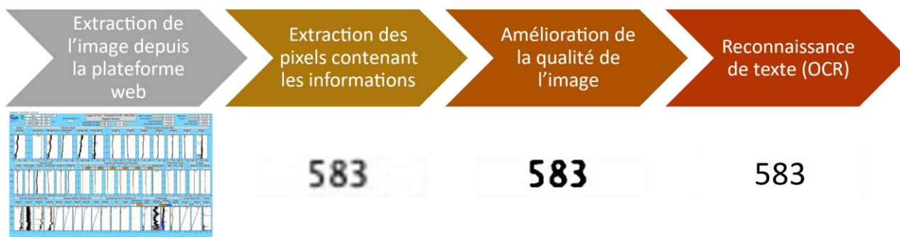
Figure 4 - Méthode d'extraction des paramètres de pilotage de tunnelier à partir d'images
