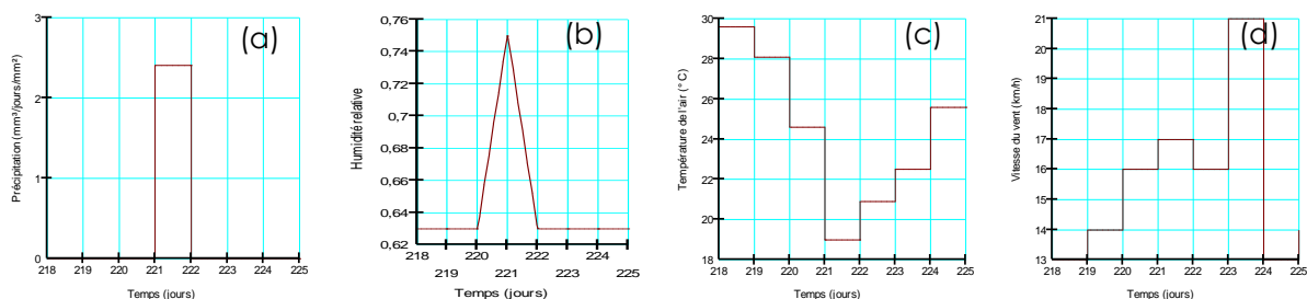
Figure 6. Conditions aux limites de la fonction climat sur Seep/w entre le 6 et le 12 août 2018 (a) précipitation (b) humidité relative (c) température moy./jour (d) vitesse du vent moy./jour.
