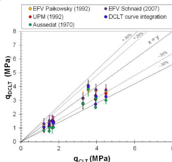
Figure 5. Comparaison des valeurs de résistances ultimes obtenues
