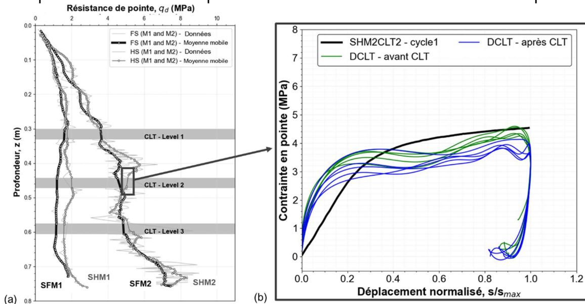
Figure 4. (a) Pénétragramme de l'éprouvette SHM2 (b) exemple de courbes de chargement (Niveau 2) : courbes DCLT avant l'essai CLT, courbe CLT et courbes DCLT après l'essai CLT
