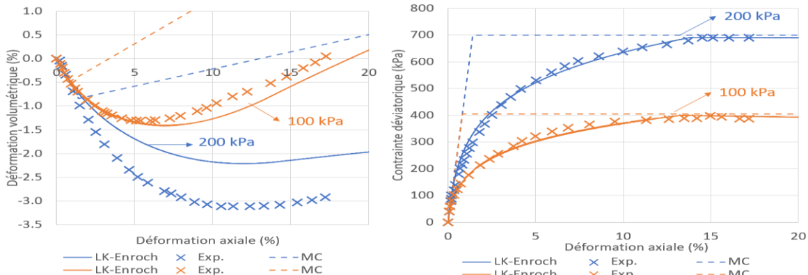
Figure 5. Expériences et simulations d'essais triaxiaux pour le remblai à l'aide des modèles MC et LK Enroch : déformation volumétrique (à gauche) et contrainte déviatorique (à droite).
