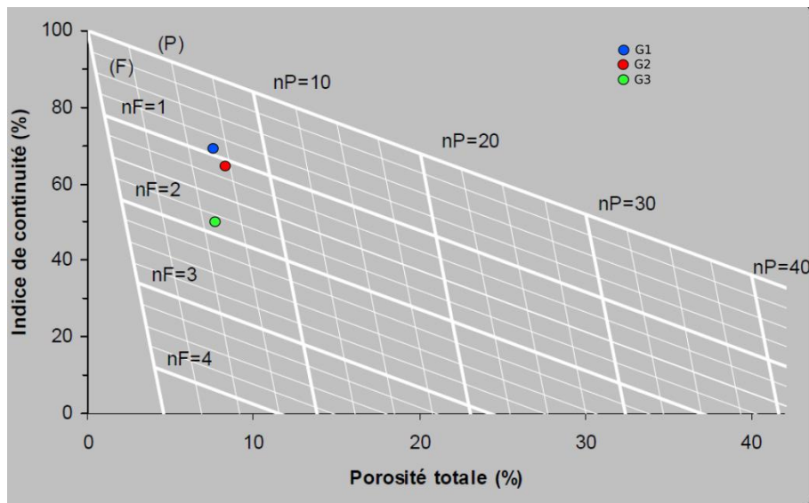
Figure 4. Evaluation par lecture du graphique de la porosité liée aux pores ( n_P en %) et de la porosité liée aux fissures ( n_F en %) à partir de l'indice de continuité qui est calculé par Eq(2) et de la porosité totale à l'eau ( N_t ) – Tourenq (1971) modifié par Saad (2011).
